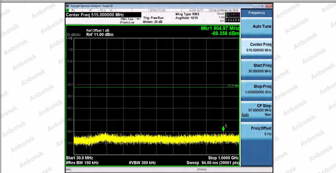
802.11n(HT20) SISO_Ant1_2412_30~1000
