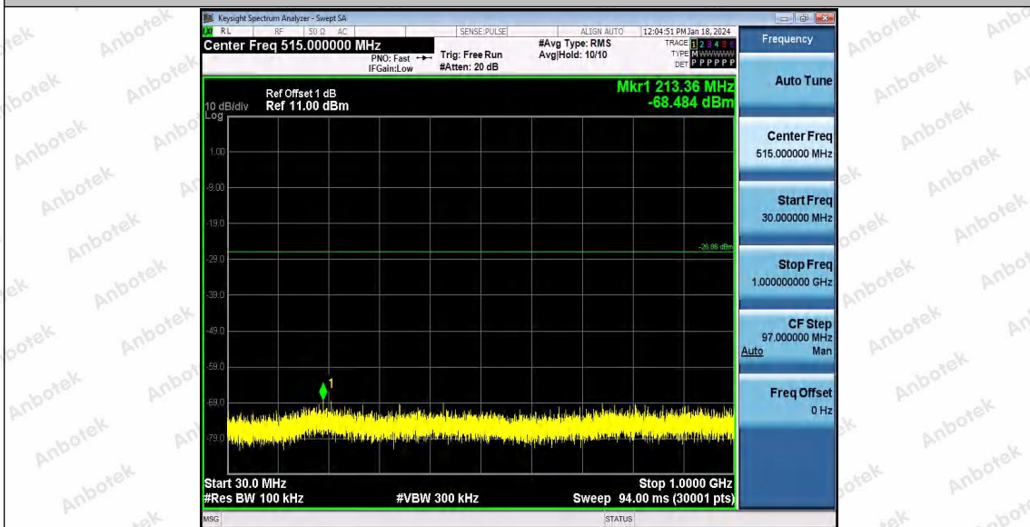
802.11b_Ant1_2437_30~1000
