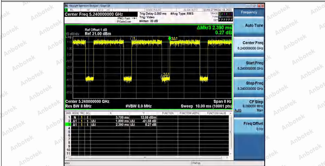
802.11n(HT20) SISO_Ant1_5240
