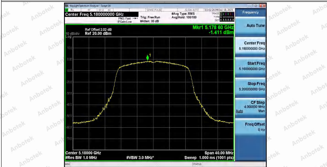
802.11n(HT20) SISO_Ant1_5180
