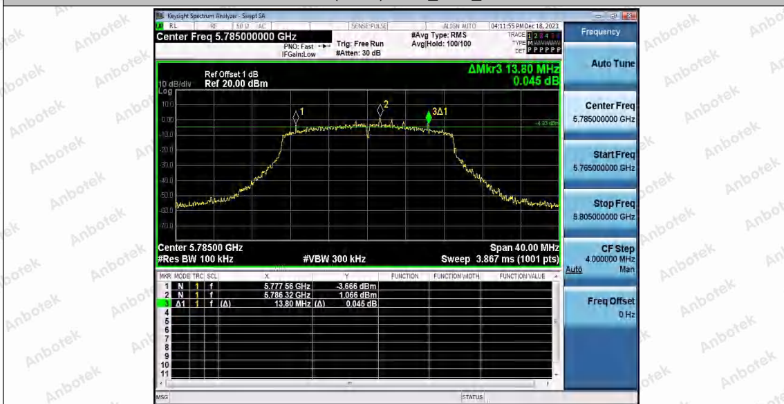
802.11n(HT20) SISO_Ant1_5785
