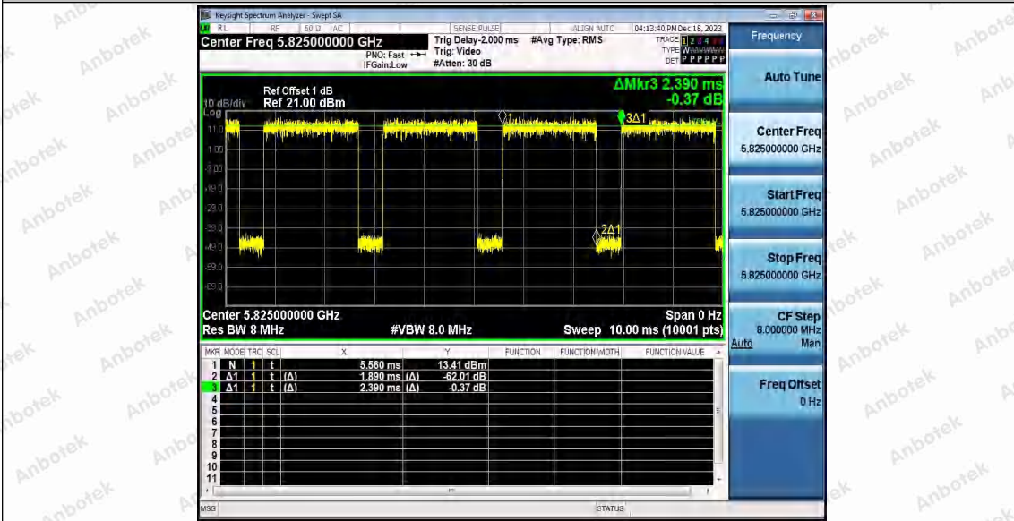
802.11n(HT20) SISO_Ant1_5825
