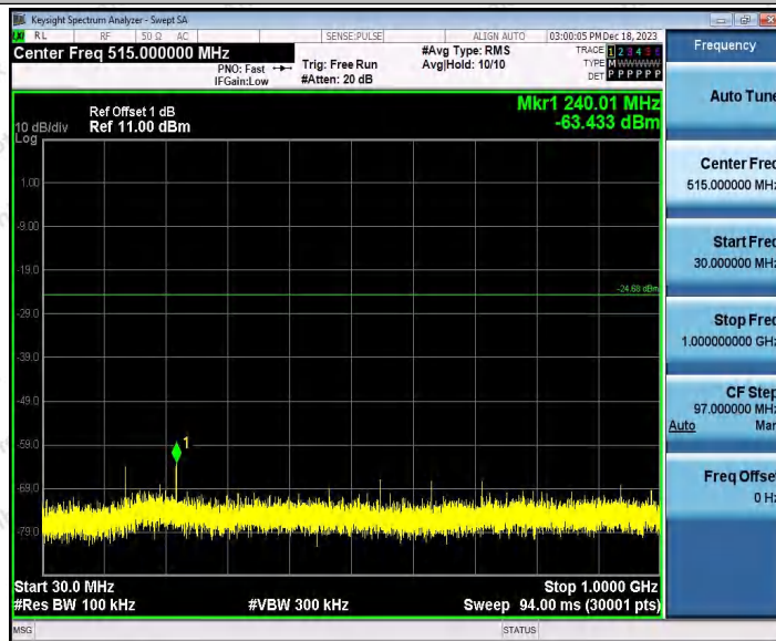
802.11b_Ant1_2437_30~1000
