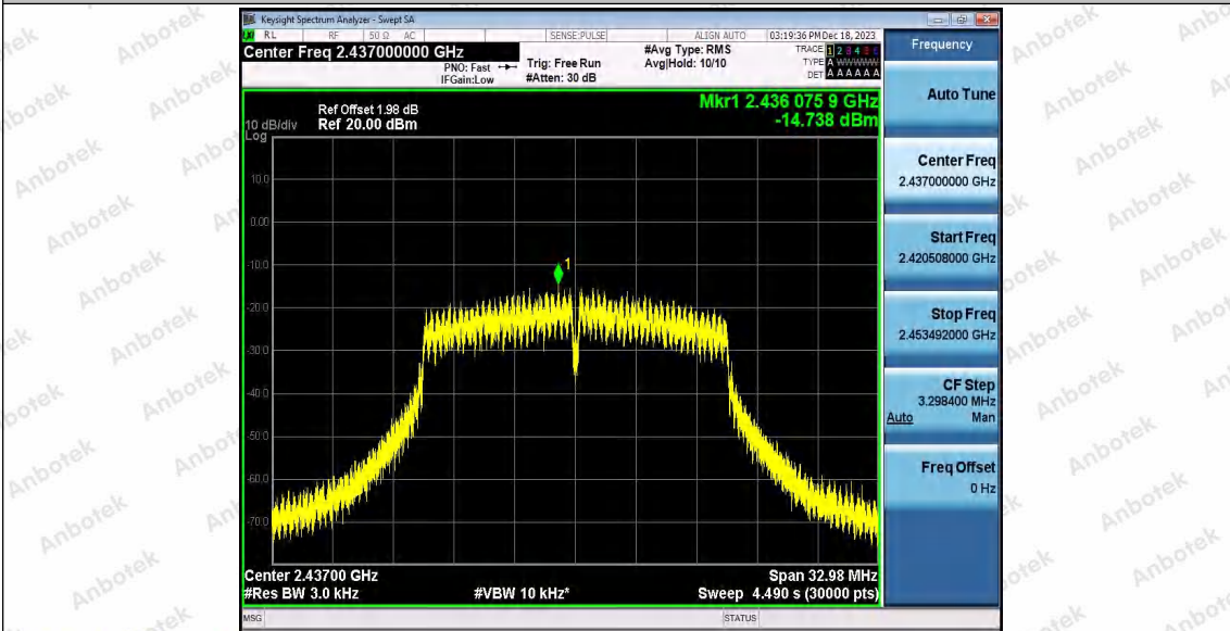
802.11g_Ant1_2437
