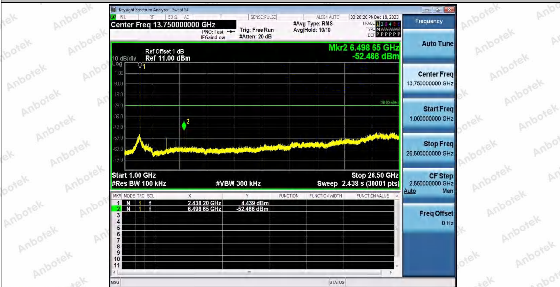
802.11g_Ant1_2437_1000~26500
