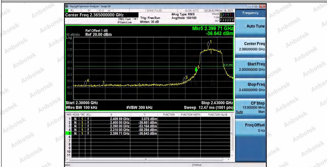
802.11n(HT20) SISO_Ant1_Low_2412
