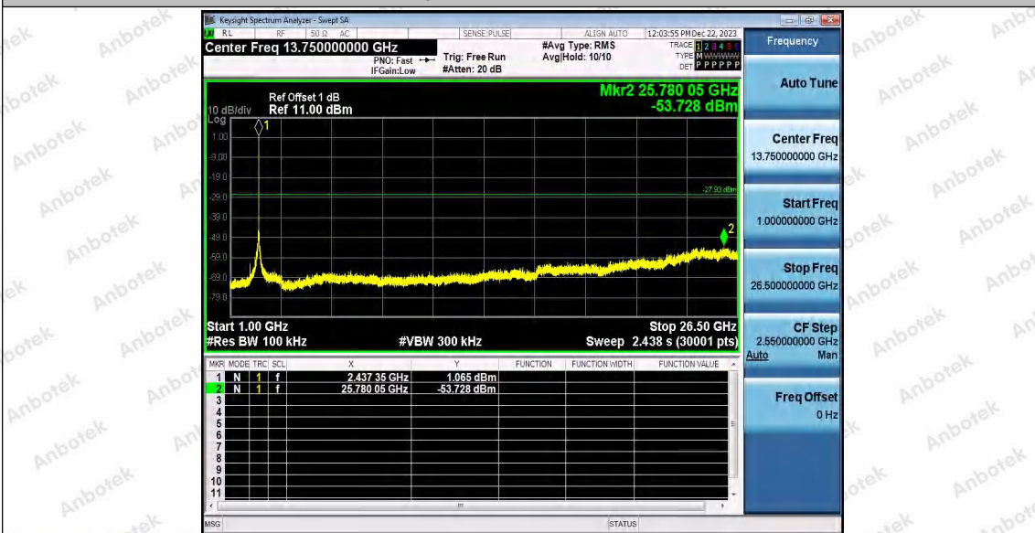
802.11g_Ant2_2437_1000~26500
