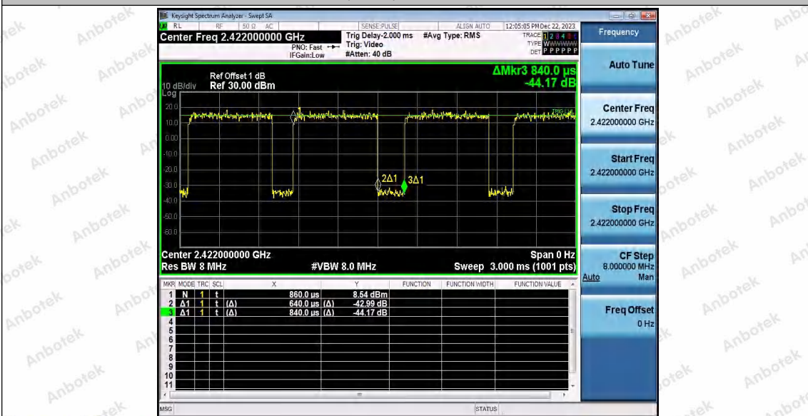
802.11n(HT40)SISO_Ant2_2422
