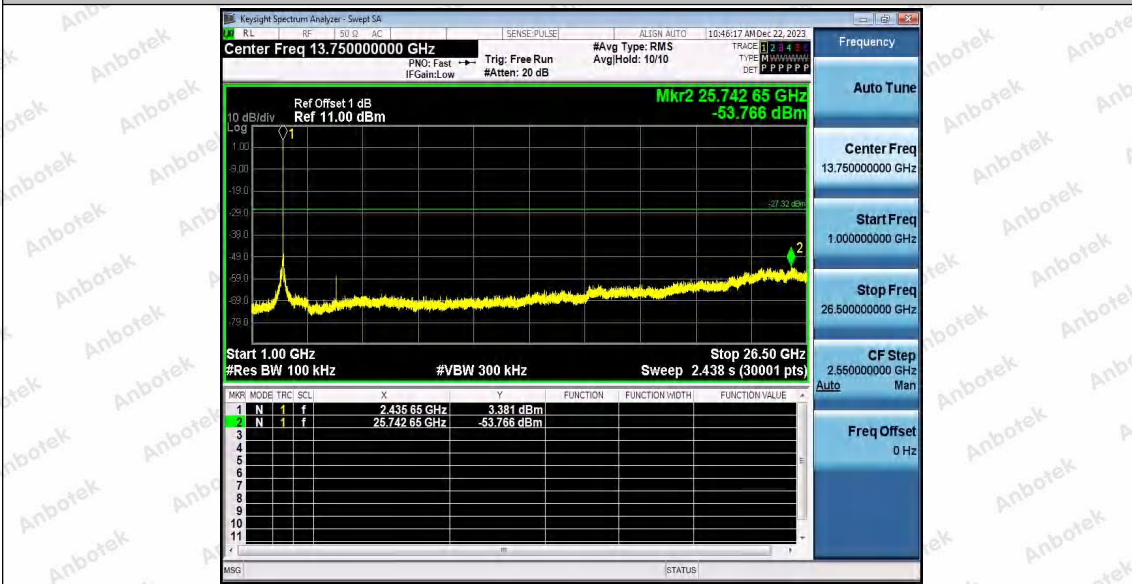
802.11b_Ant2_2437_0~Reference
