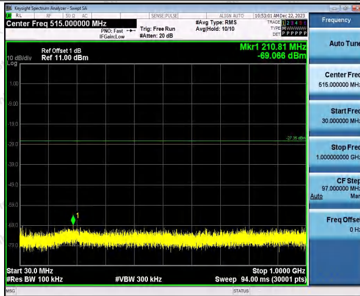
802.11g_Ant1_2412_30~1000
