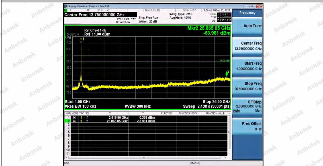
802.11n(HT40)SISO_Ant2_2422_1000~26500
