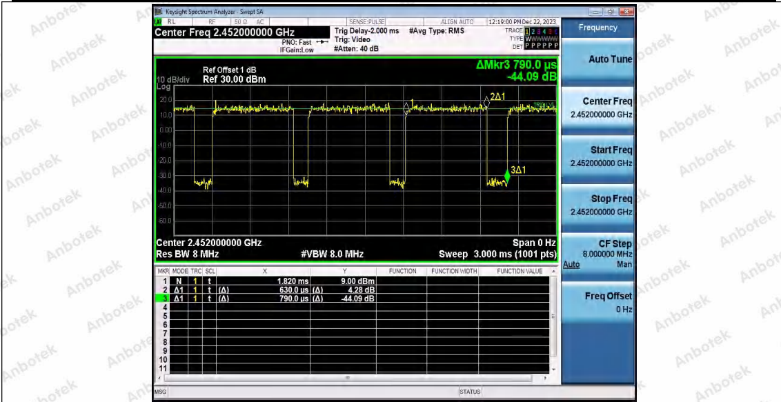
802.11n(HT40)SISO_Ant2_2452
