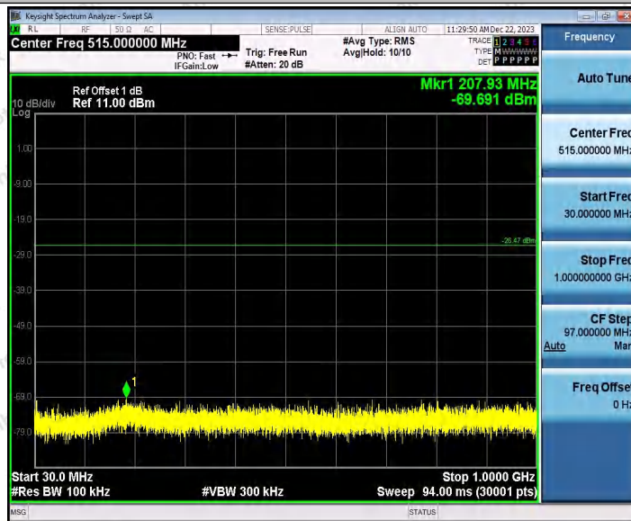
802.11b_Ant2_2412_30~1000
