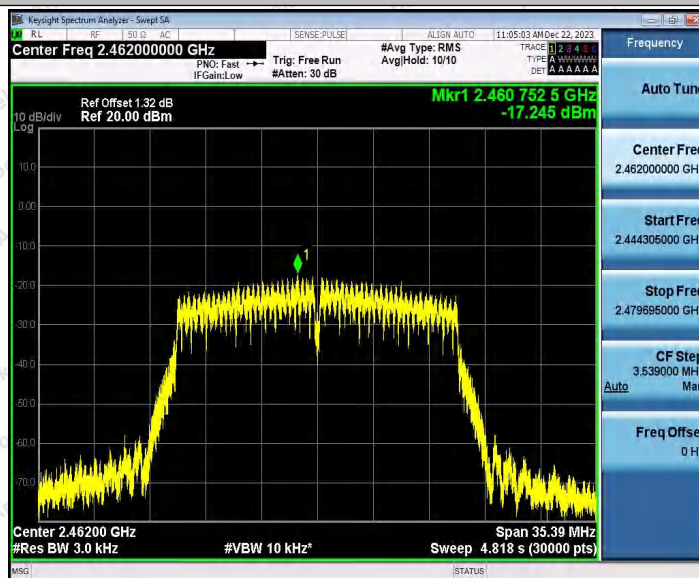
802.11n(HT20)SISO_Ant2_2462
