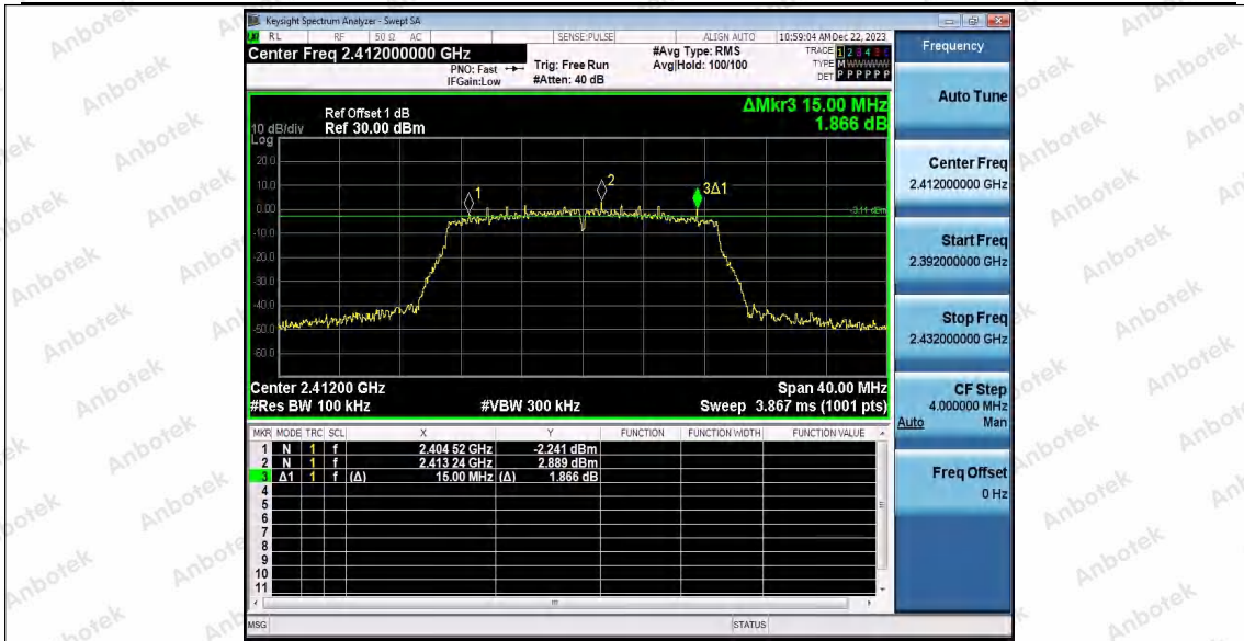
802.11n(HT20)SISO_Ant2_2412
