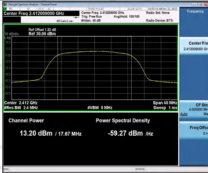
802.11n(HT20)SISO_Ant2_2412
