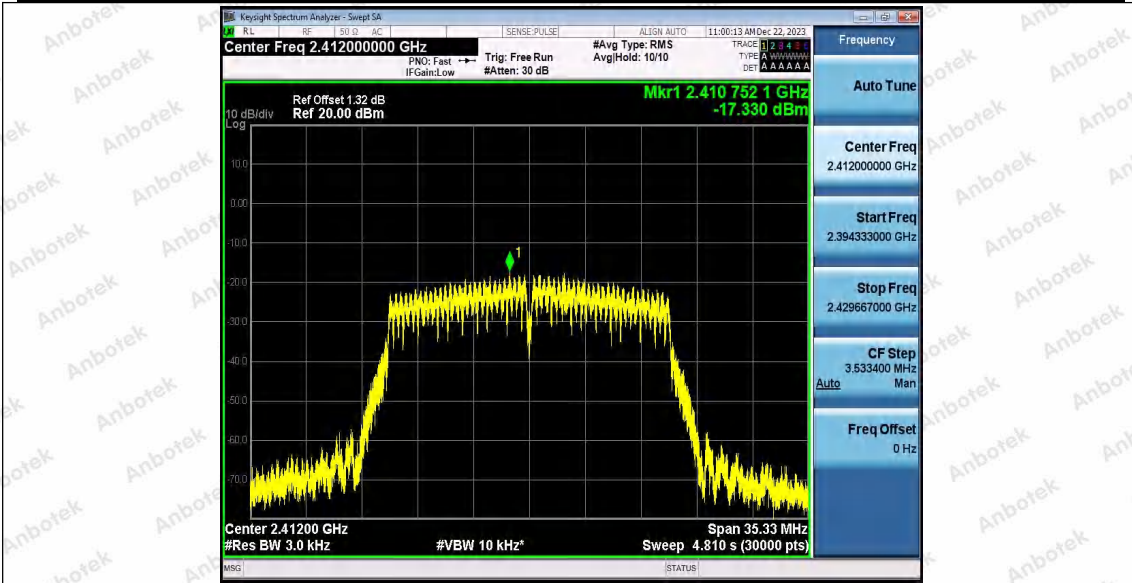
802.11n(HT20)SISO_Ant2_2412
