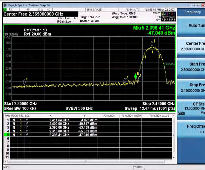
802.11b_Ant2_Low_2412
