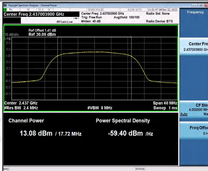
802.11n(HT20)SISO_Ant1_2437
