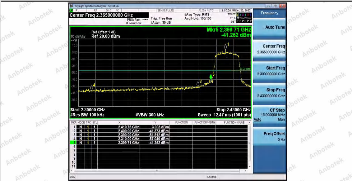
802.11n(HT20)SISO_Ant2_Low_2412
