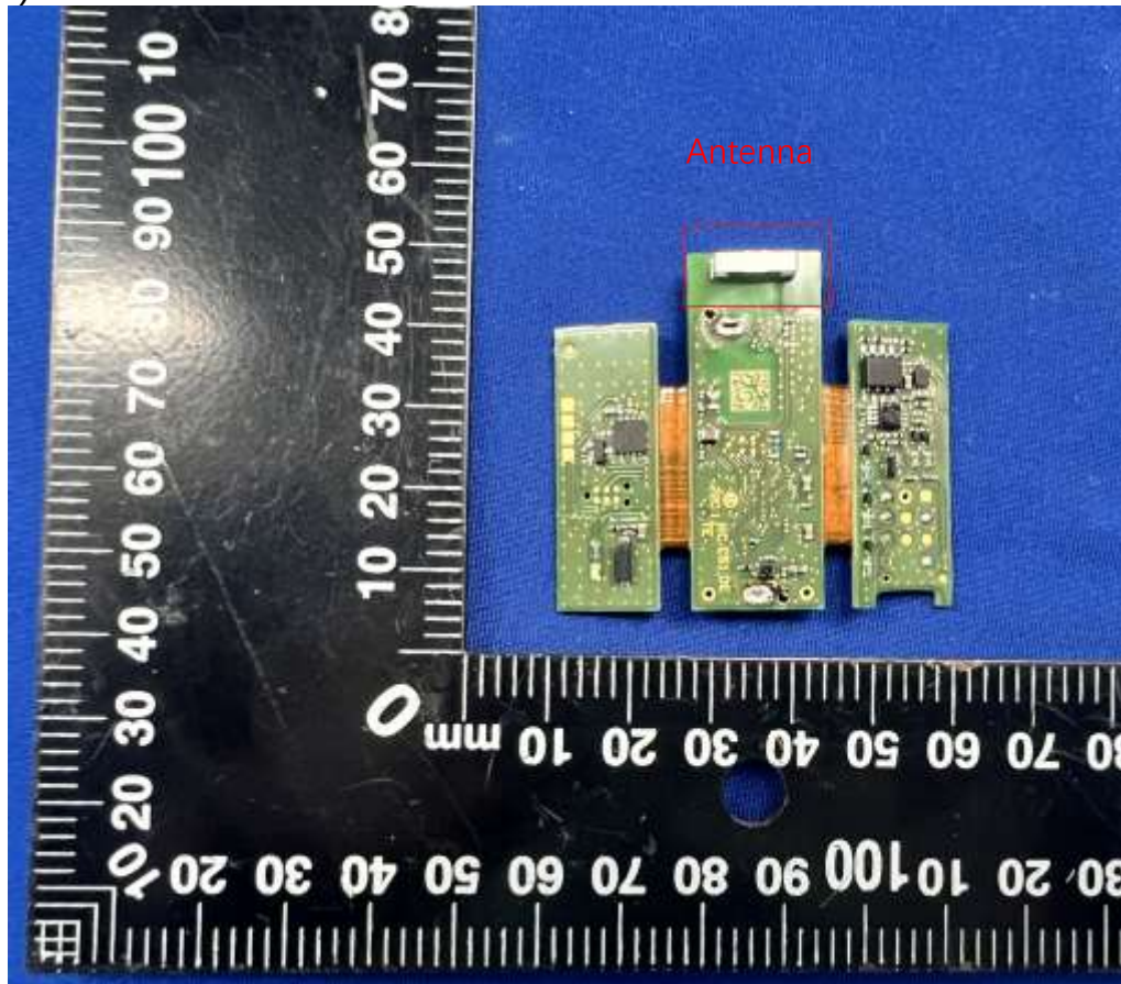
6) EUT Photo
