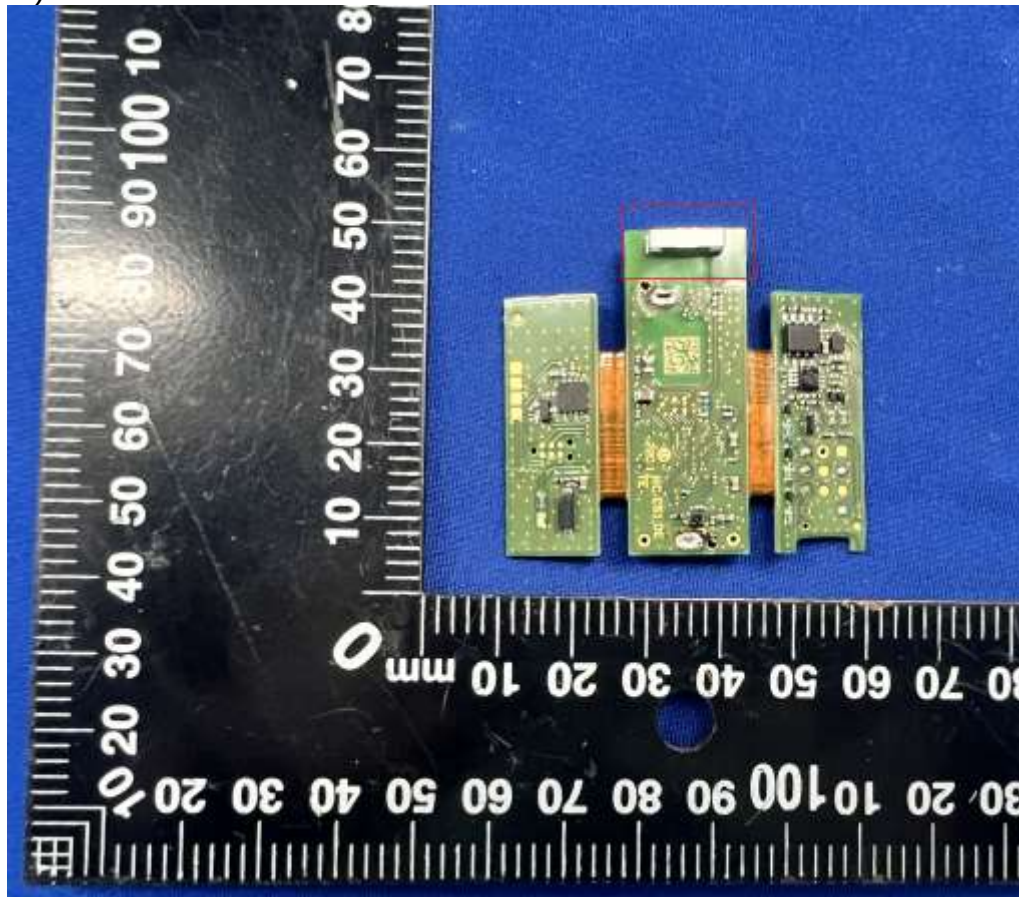
14) EUT Photo
