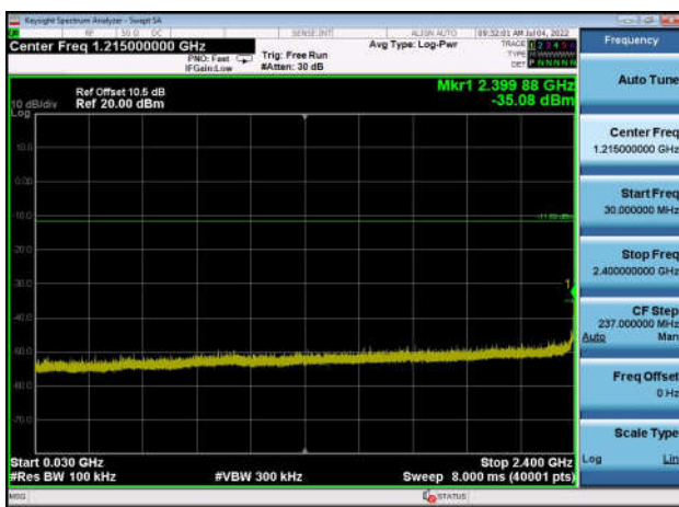
,Plot 3,30MHz~2400MHz-802.11b,2462MHz ,Ant0
