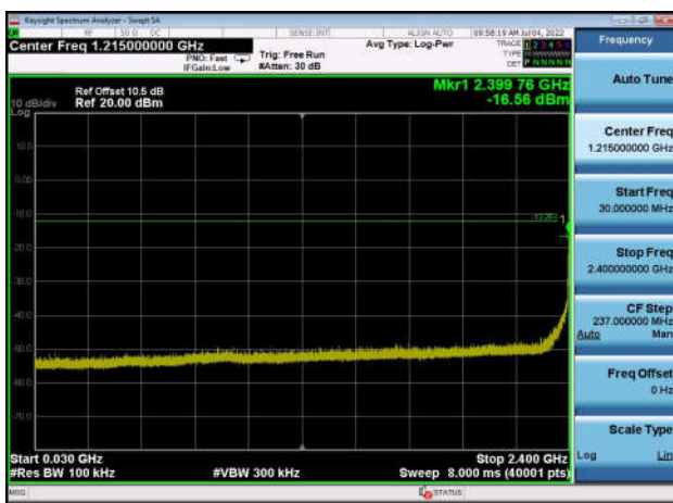
,Plot 3,30MHz~2400MHz-802.11g,2462MHz ,Ant0
