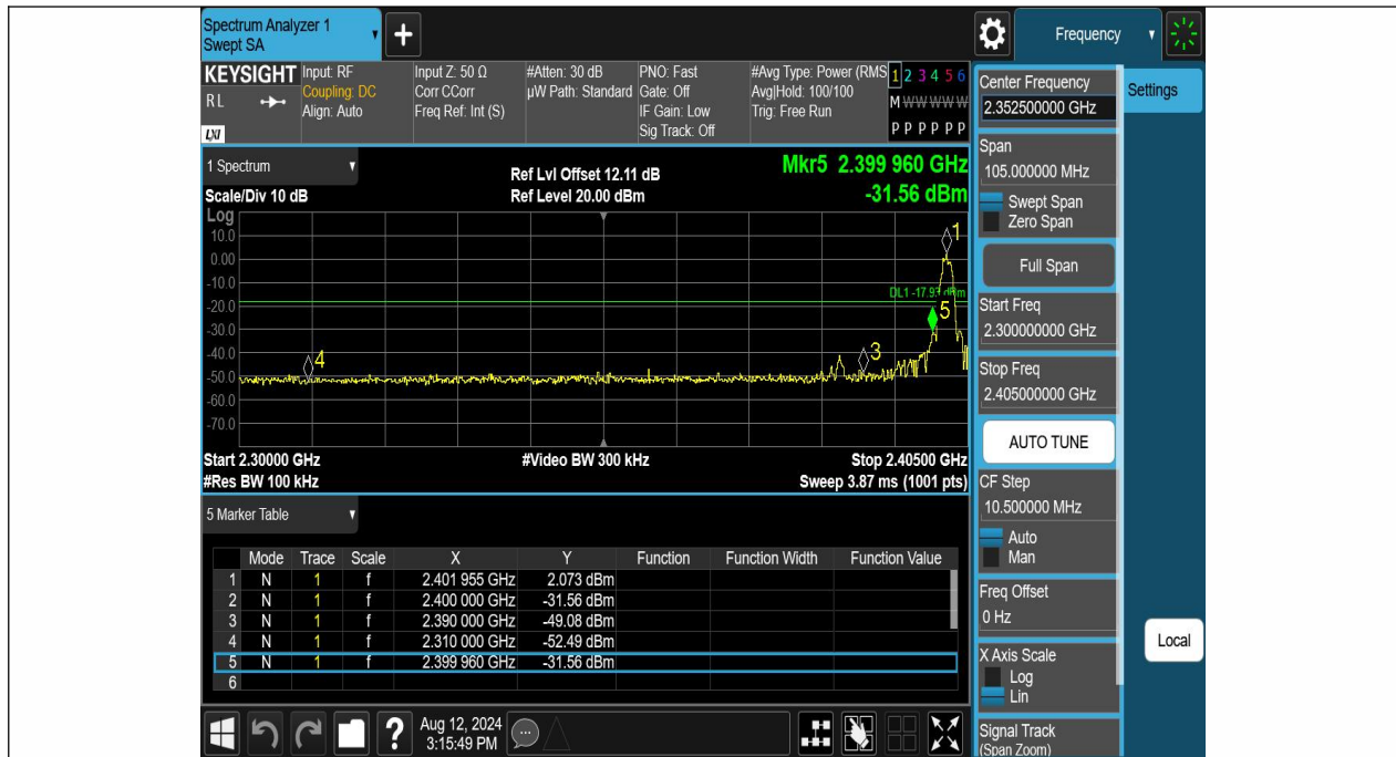
BLE 2M-Ant1-2402-PASS
