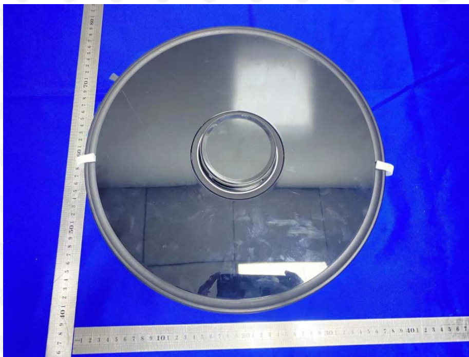
EUT Photo 2
