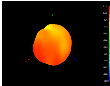
2450MHz
