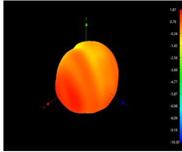
2400MHz
