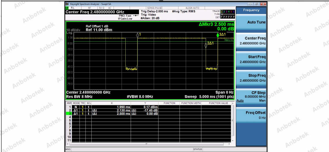
NTNV-BLE 1M-Ant1-2480
