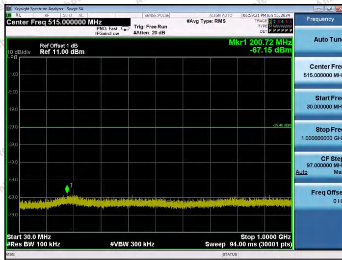
11G-Ant1-2412-30~1000-PASS
