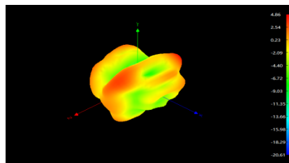
2450MHz
