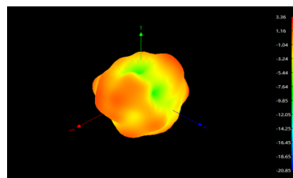
2400MHz
