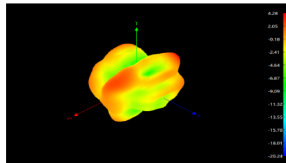
2500MHz
