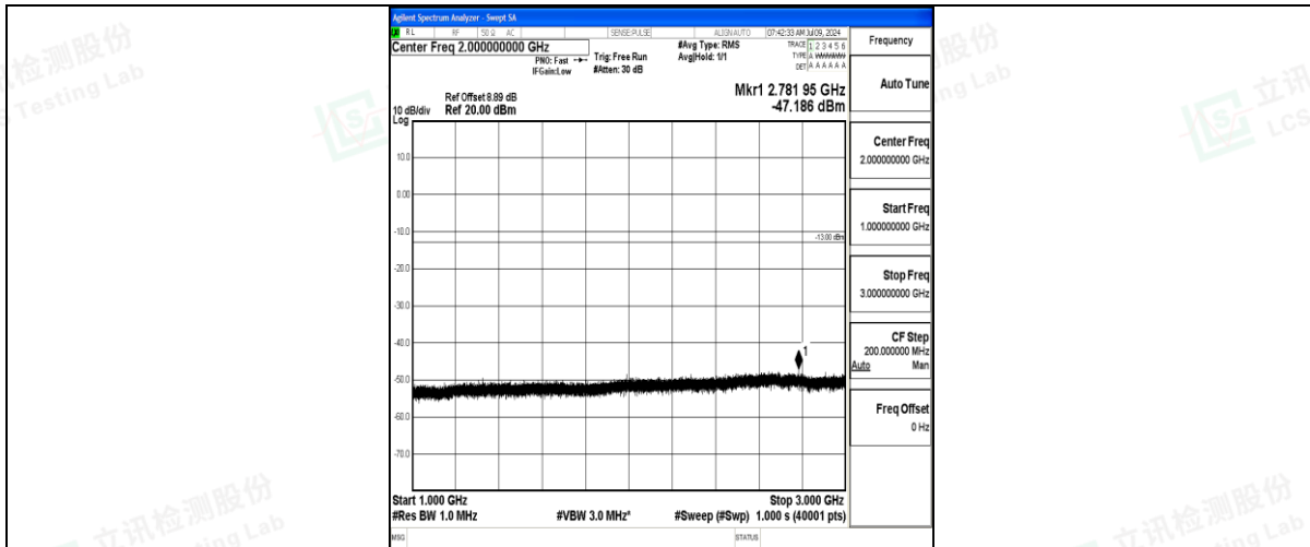
Band71_10MHz_QPSK_133172_1RB#0_1000~3000_1000~3000
