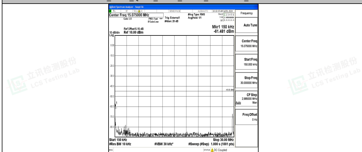
Band41 5MHz QPSK 40620 1RB#0 0.15~30 0.15~30
