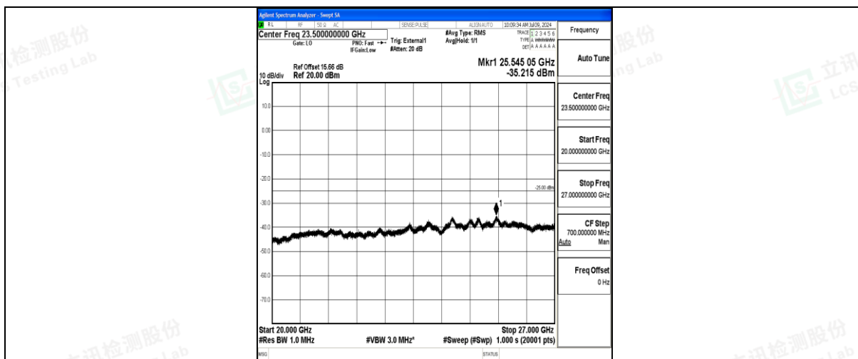
Band41 5MHz 16QAM 39675 1RB#0 20000~27000 20000~27000
