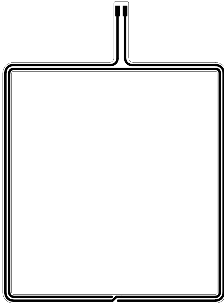
Fig. 4.1.5 RFID Antenna layout
