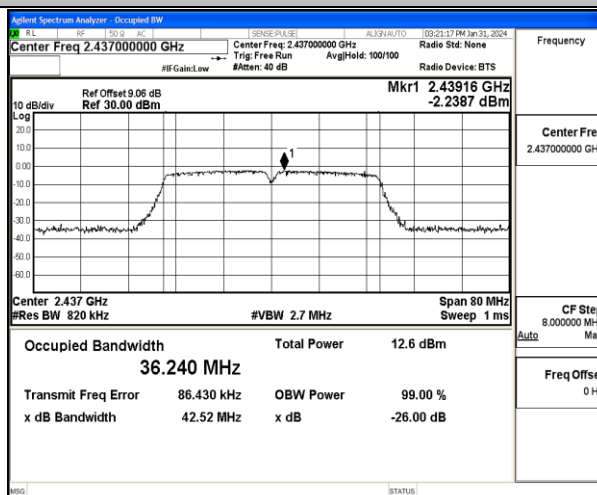
11N40MIMO-Ant1-2437
