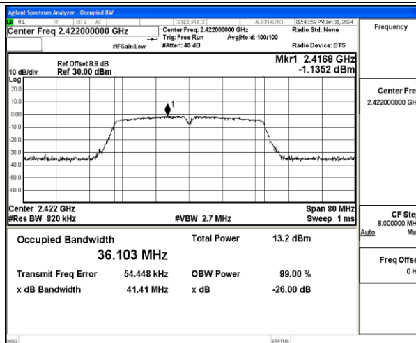
11N40MIMO-Ant1-2422
