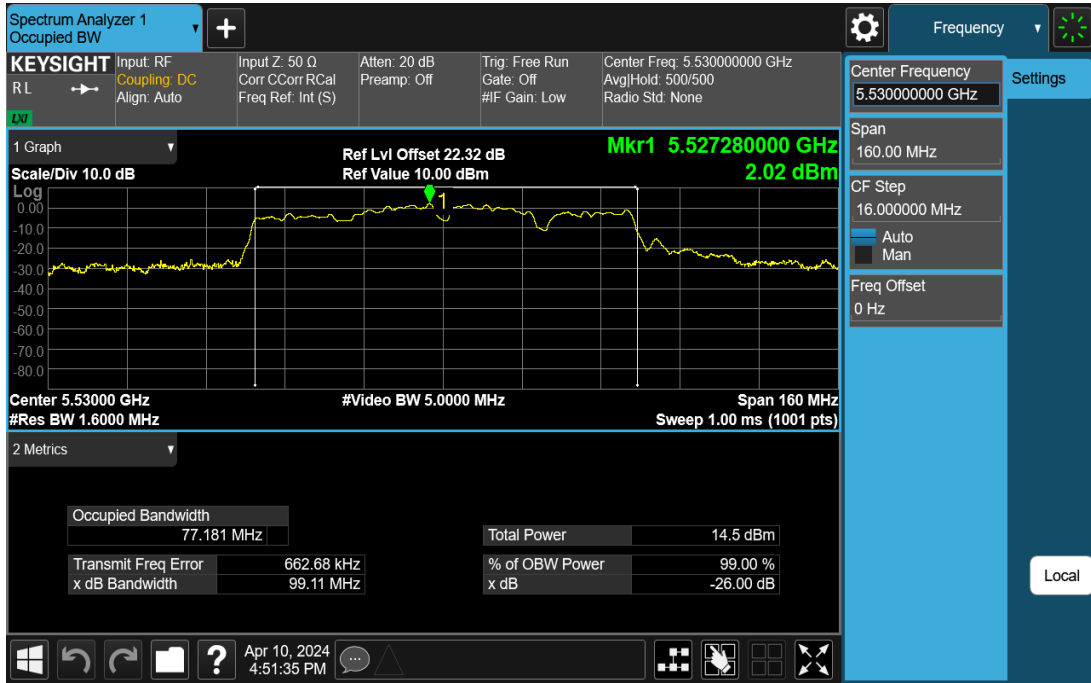
11AC80SISO-Ant1-5530
