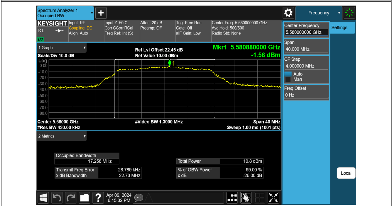
11A-Ant1-5580
