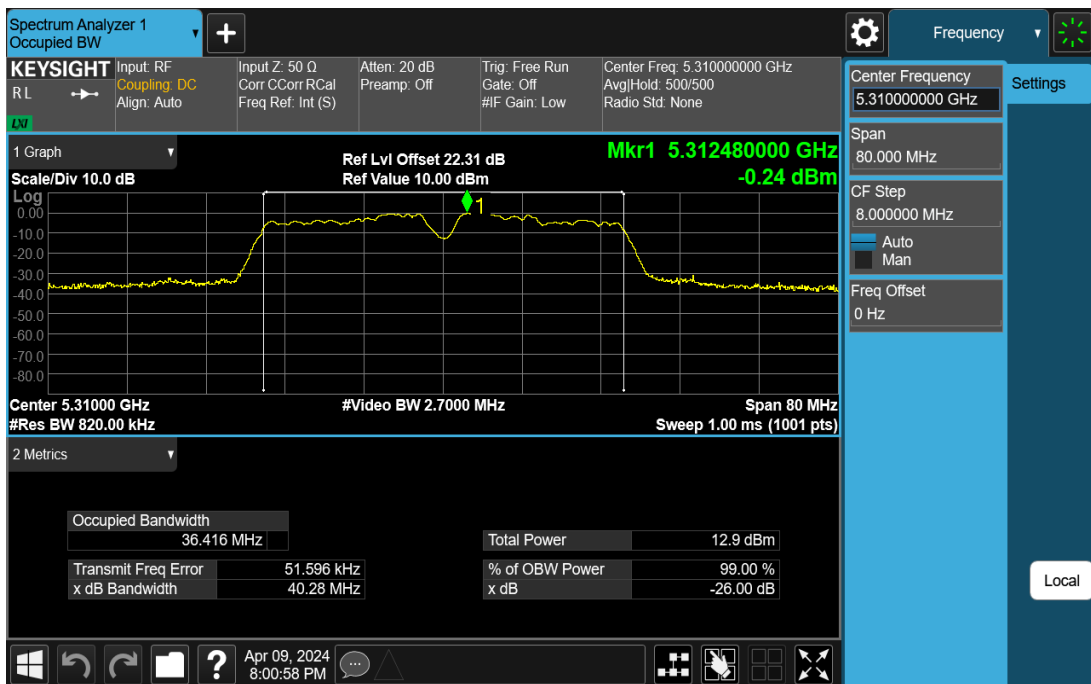
11N40SISO-Ant1-5310
