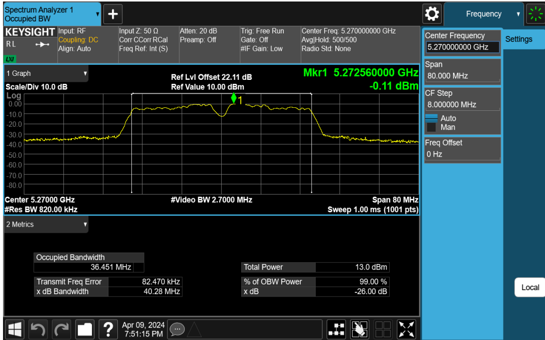
11N40SISO-Ant1-5270
