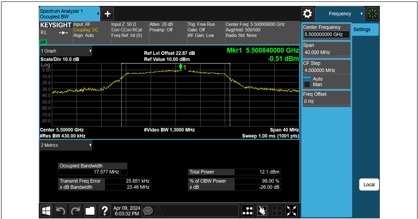
11A-Ant1-5500
