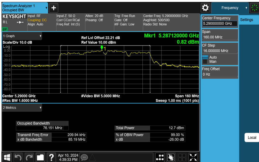
11AC80SISO-Ant1-5290
