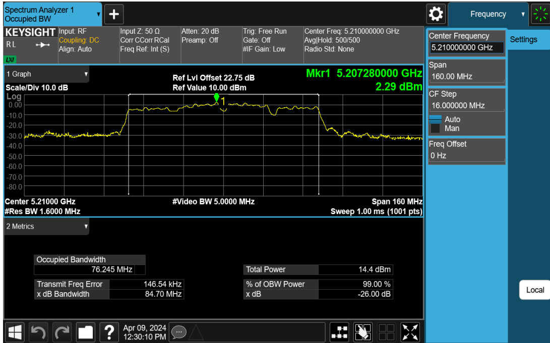
11AC80SISO-Ant1-5210
