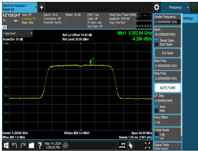
11N20MIMO-Ant1-5200-PASS
