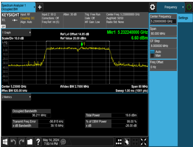
11N40MIMO-Ant2-5230
