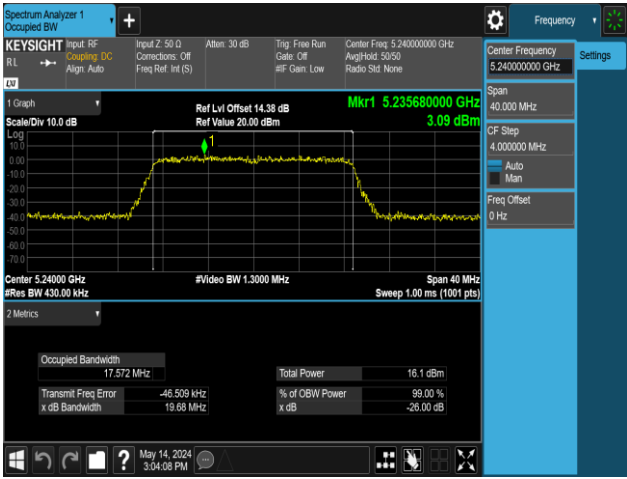
11N20MIMO-Ant1-5240
