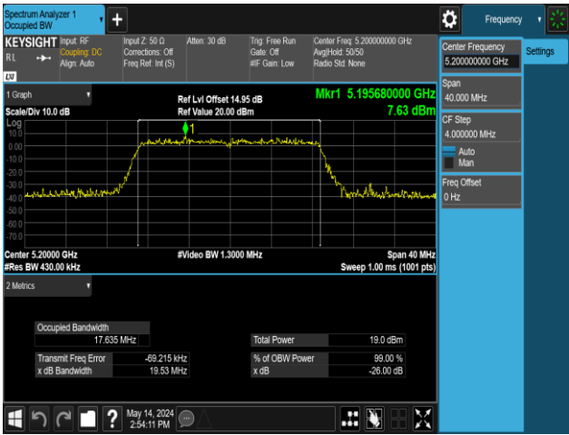
11N20MIMO-Ant2-5200
