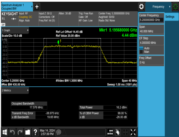
11N20MIMO-Ant1-5200
