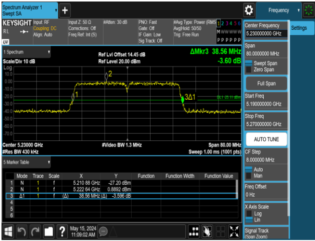
11AC40MIMO-Ant1-5230
