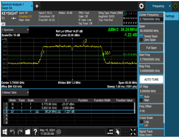
11AC40MIMO-Ant1-5795
