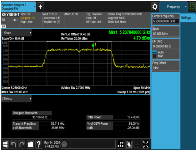
11N40MIMO-Ant1-5230
