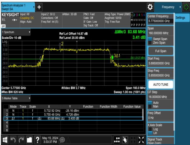
11AC80MIMO-Ant1-5775
