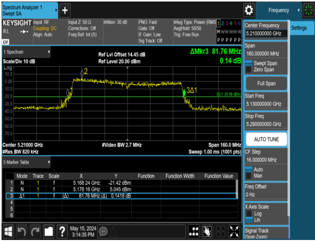
11AC80MIMO-Ant1-5210
