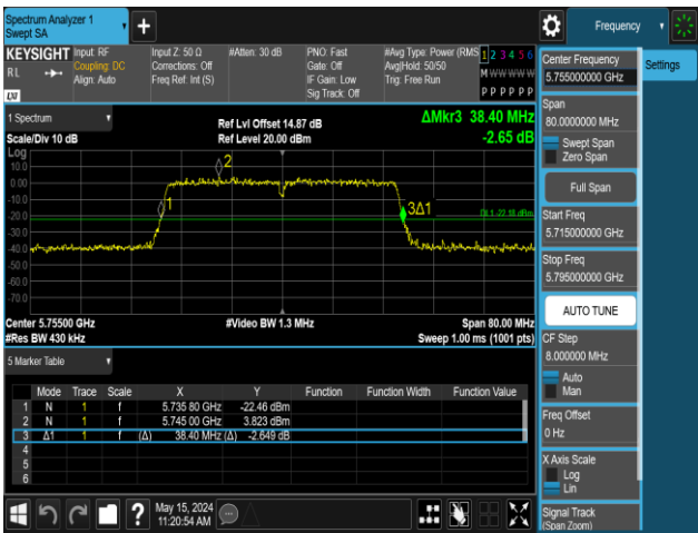
11AC40MIMO-Ant1-5755
