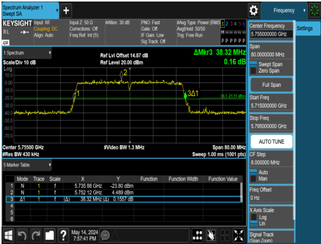
11N40MIMO-Ant1-5755
