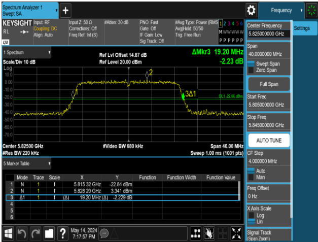
11N20MIMO-Ant1-5825
