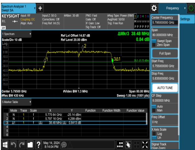
11N40MIMO-Ant1-5795
