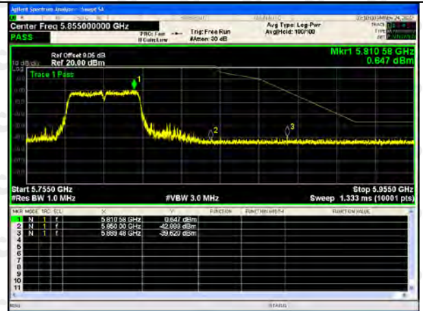
802.11ac(VH20)-5825
