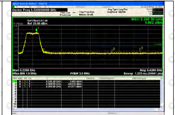
802.11n(HT40)-5230
