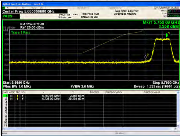
802.11(n40)-5755
