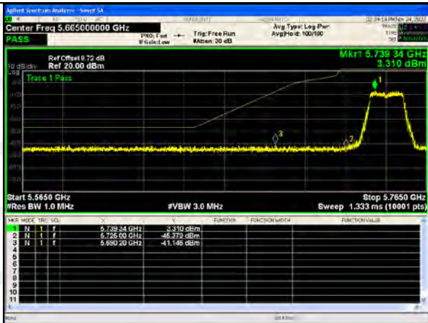
802.11(n20)-5745
