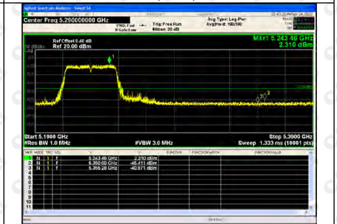
802.11n(HT40)-5230
