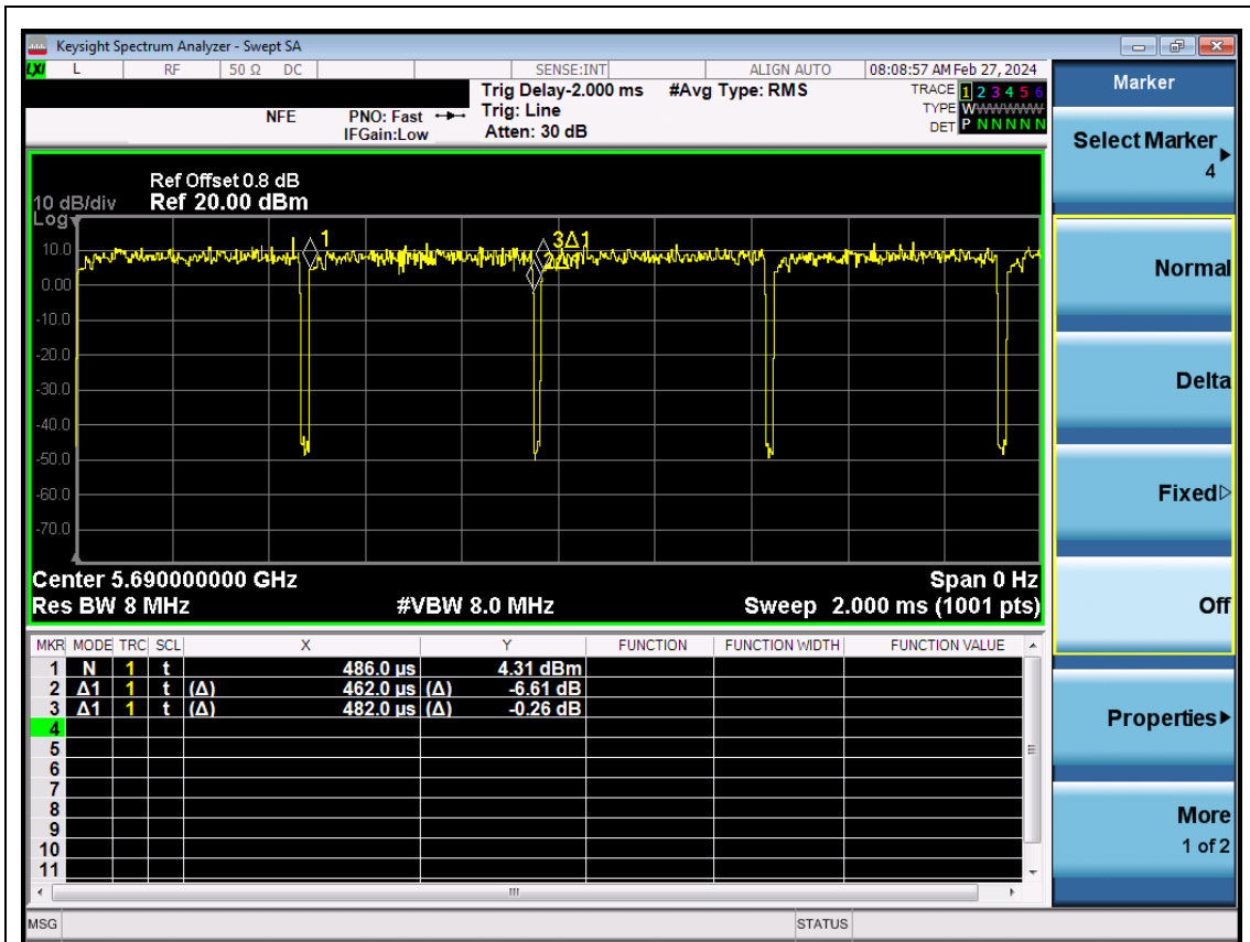
NTNV-11AC80SISO-Ant1-5690
