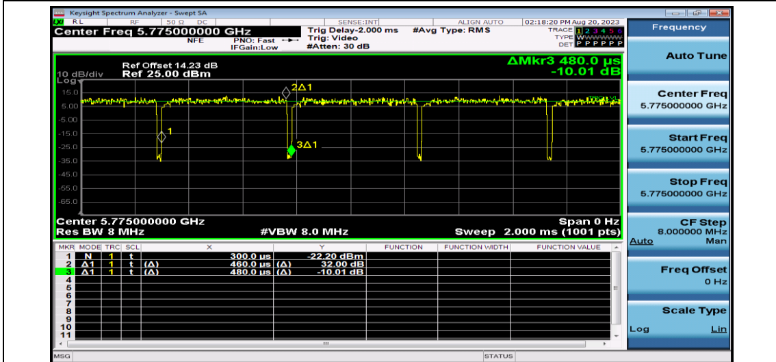
NTNV-11AC80SISO-Ant1-5775
