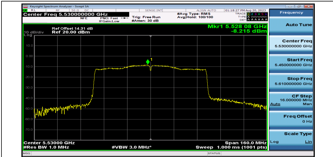
11AC80SISO-Ant1-5530
