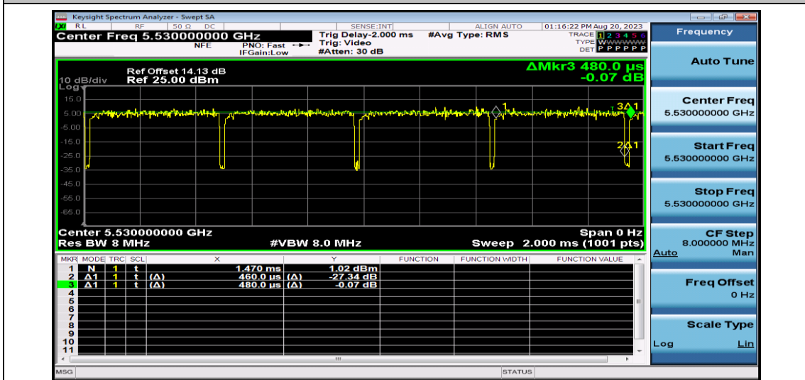
NTNV-11AC80SISO-Ant1-5530
