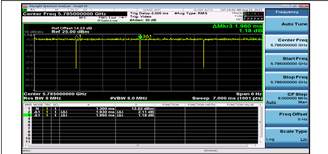
NTV-11AC20SISO-Ant1-5785
