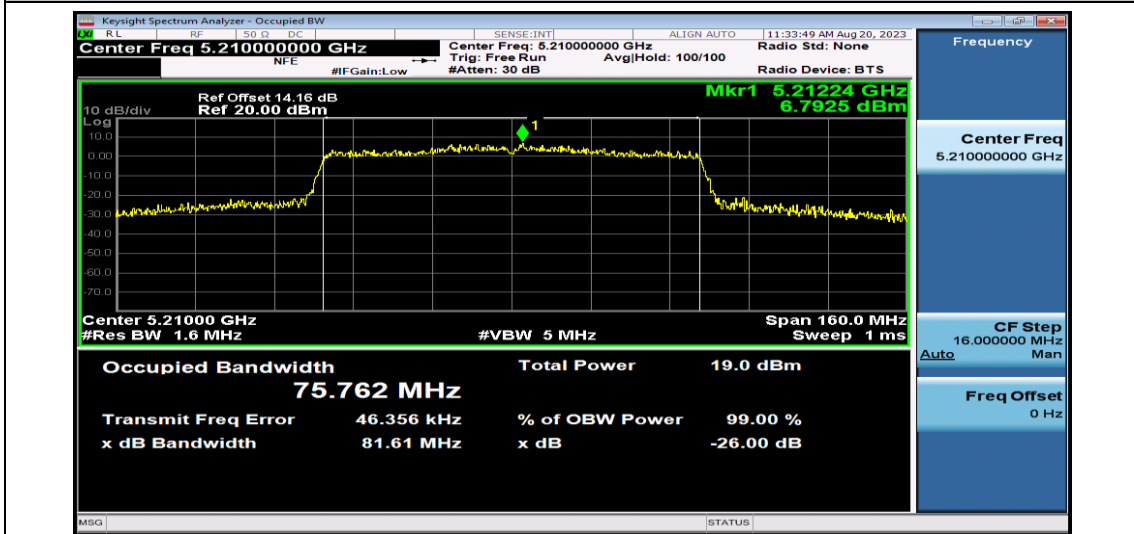
11AC80SISO-Ant1-5210
