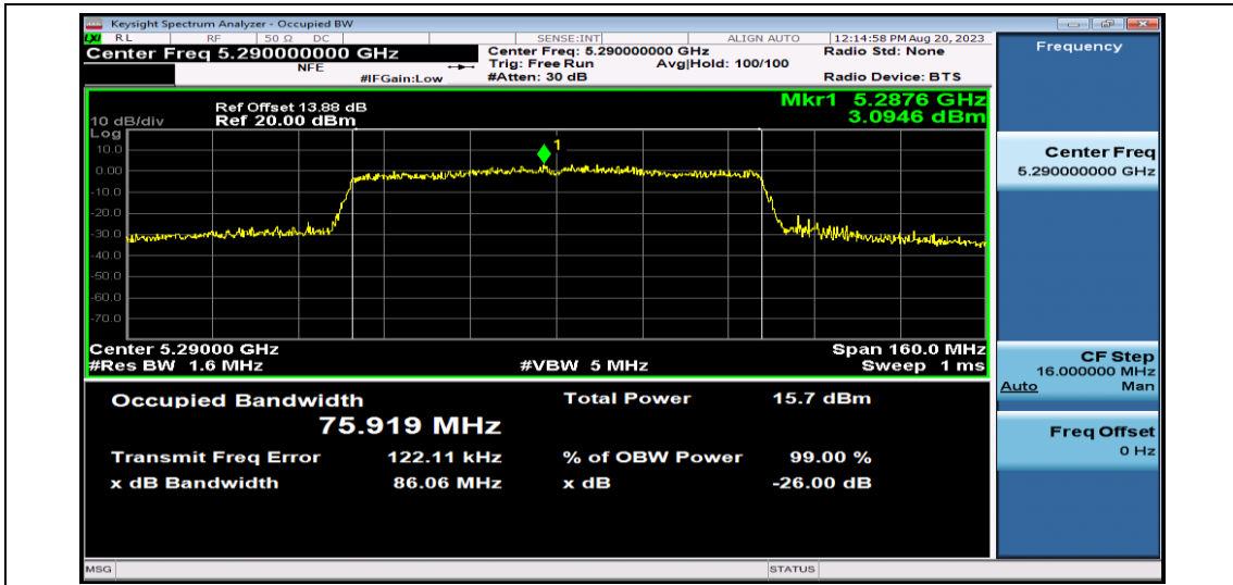
11AC80SISO-Ant1-5290
