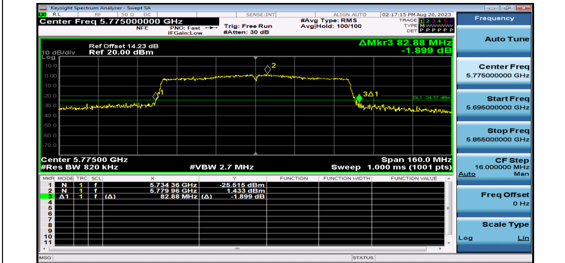
11AC80SISO-Ant1-5775
