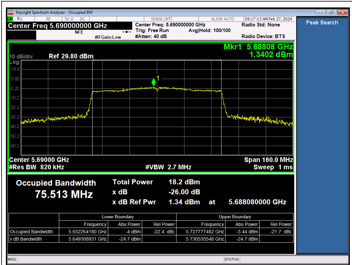
11AC80SISO-Ant1-5690
