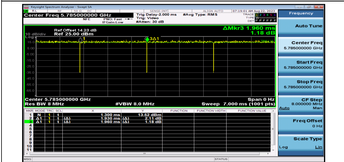
NTV-11AC20SISO-Ant1-5785
