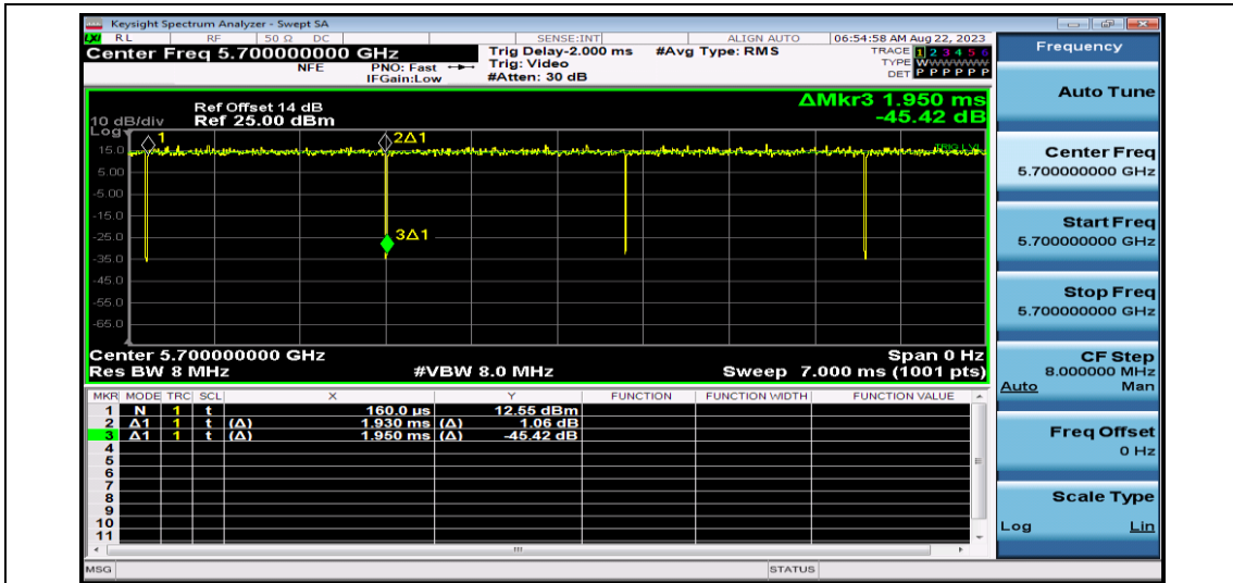
NTV-11AC20SISO-Ant1-5700
