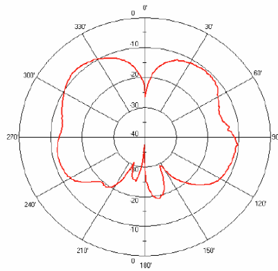
2.4 GHz H-Plane Vertical
