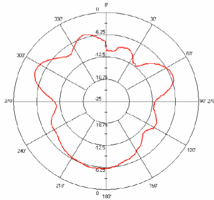
2.4 GHz H-Plane Vertical
