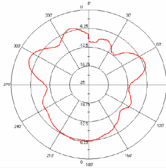
2.4 GHz H-Plane Vertical
