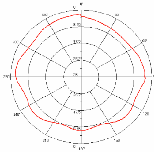
2.4 GHz H-Plane Horizontal
