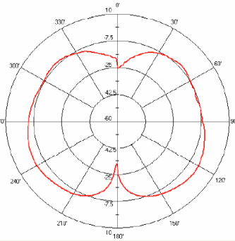
2.4 GHz H-Plane Horizontal
