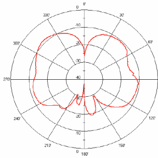
2.4 GHz H-Plane Vertical
