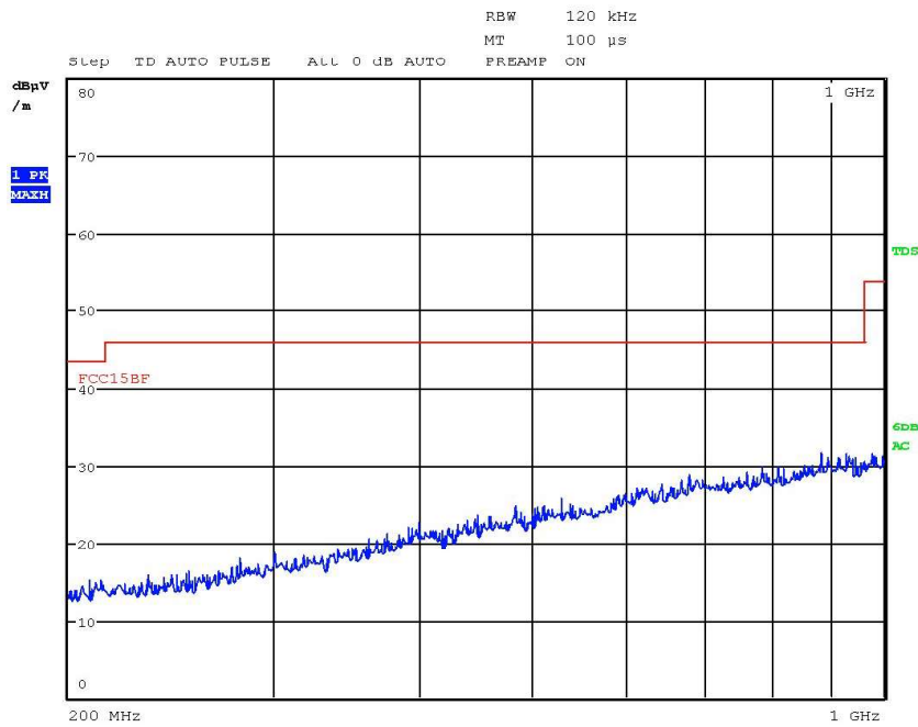
200MHz~1000MHz Vertical
