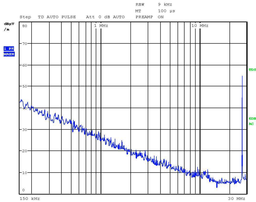
150kHz~30MHz Face
