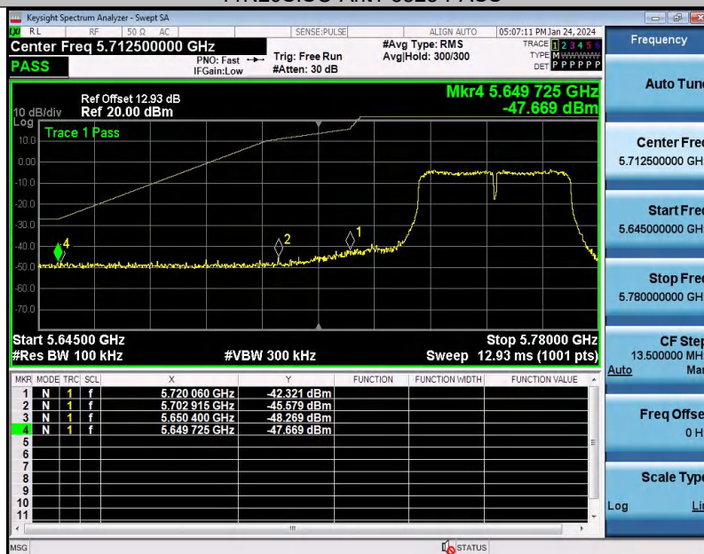
11N40SISO-Ant1-5755-PASS
