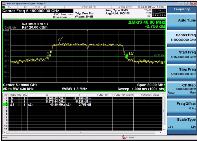
802.11n(HT40)
