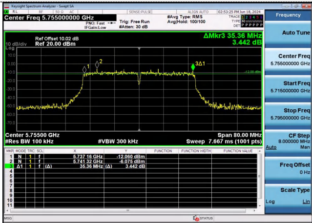
802.11ac(VHT40)
