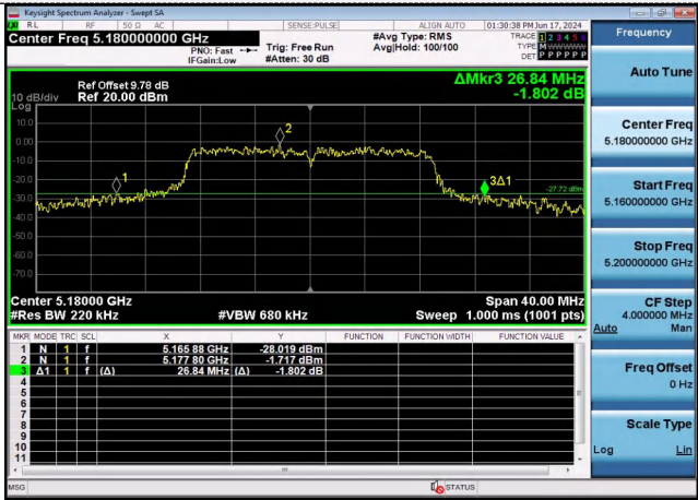
802.11ac(VHT20)
