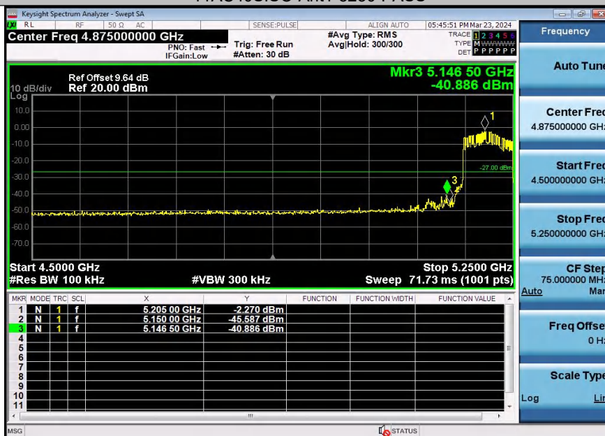
11AC80SISO-Ant1-5210-PASS
