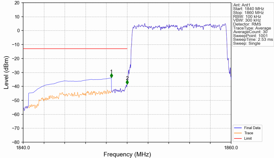
Band2_10MHz_QPSK_LCH_1855MHz_RB_50_0_NTNV
