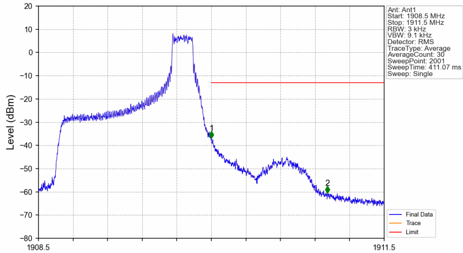
Band2_1.4MHz_QPSK_HCH_1909.3MHz_RB_1_5_NTNV
