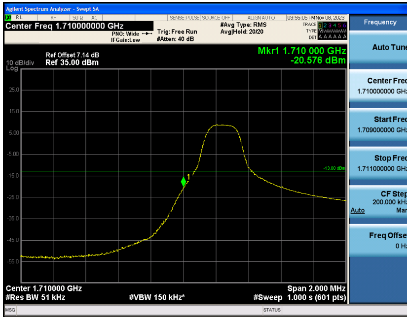
Band4-3MHz-QPSK-19965-1RB#14
