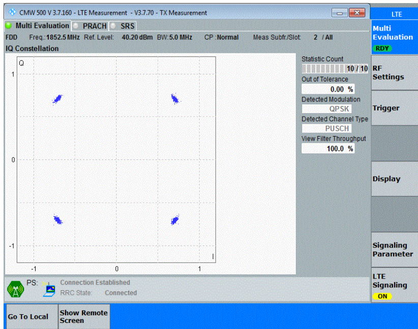
Band2-5MHz-QPSK-18900-25RB#0
