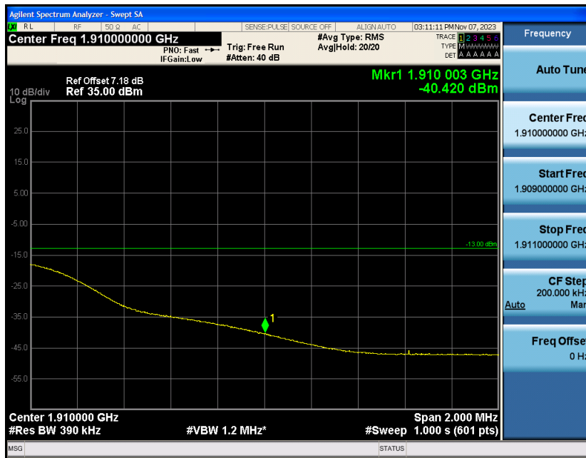
Band2-20MHz-16QAM-19100-1RB#99
