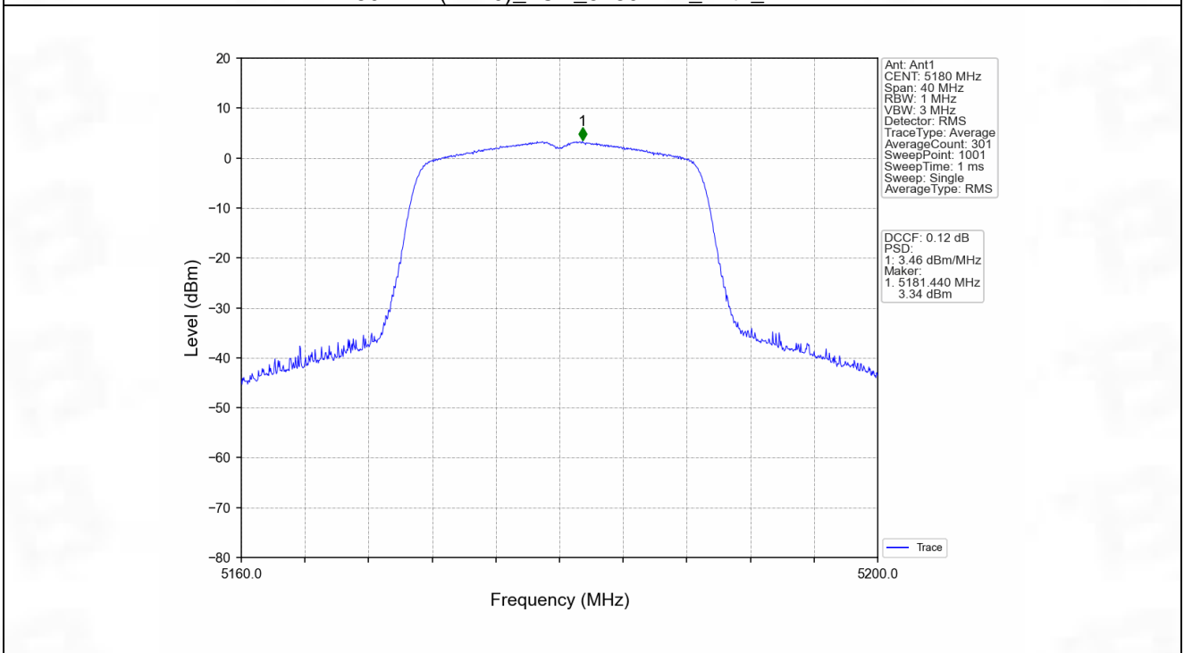
802.11n(HT20)_LCH_5180MHz_Ant1_NTNV
