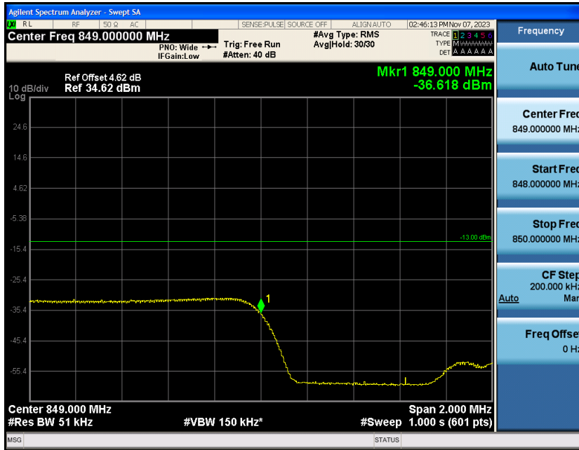
Band5-3MHz-QPSK-20635-1RB#14
