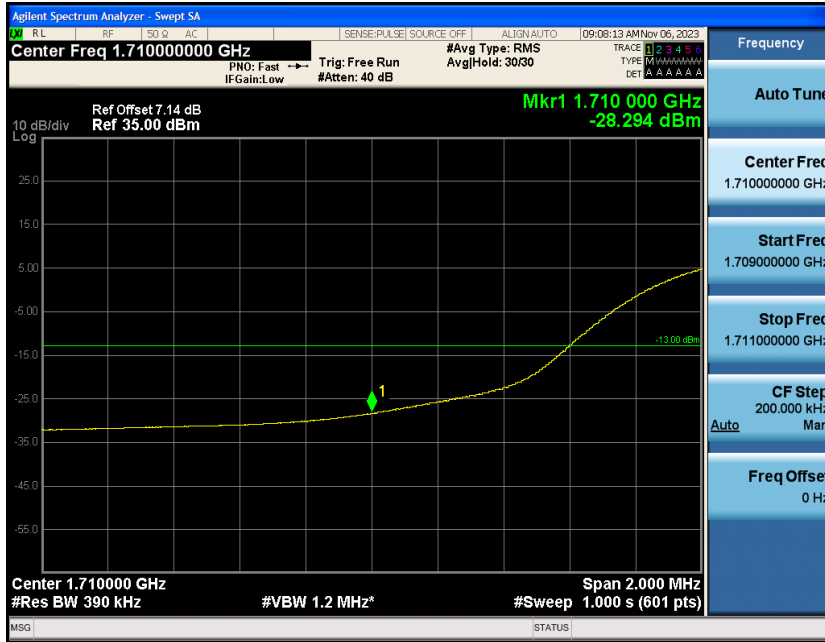
Band4-20MHz-QPSK-20050-1RB#99
