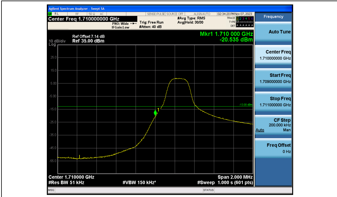
Band4-3MHz-QPSK-19965-1RB#14
