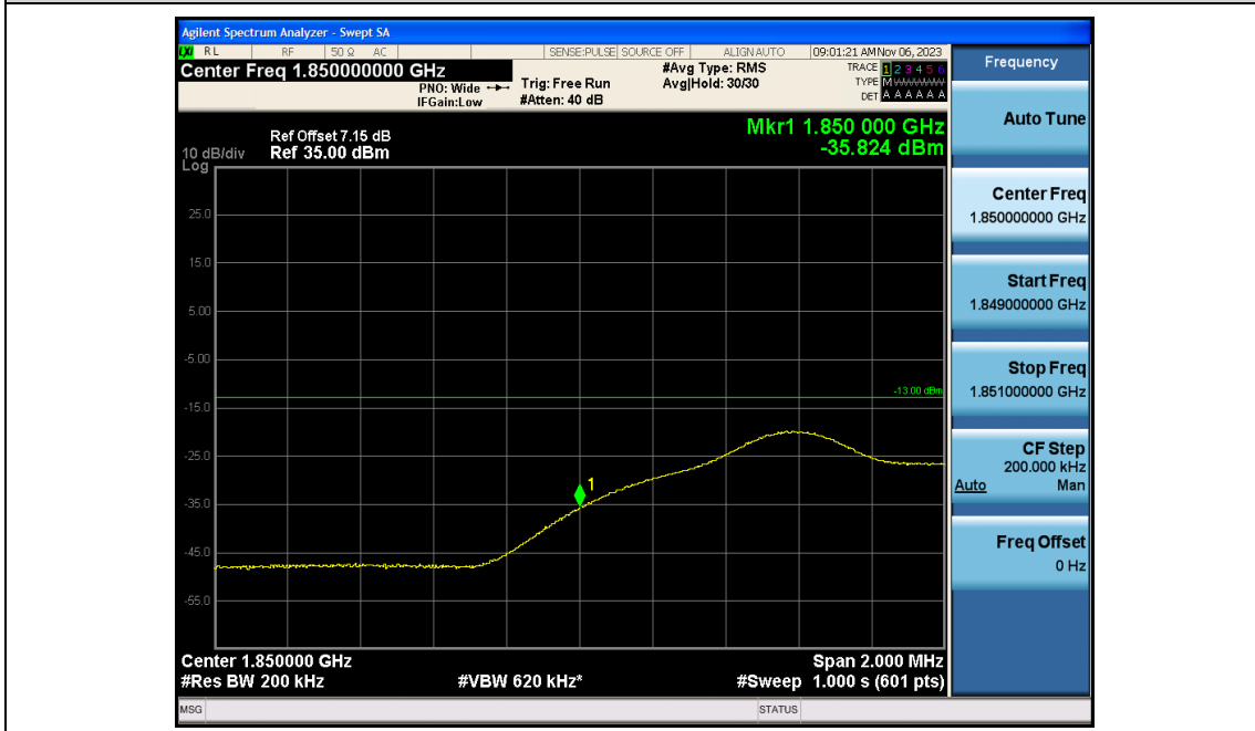
Band2-10MHz-QPSK-18650-50RB#0
