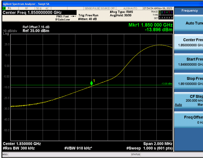
Band2-15MHz-16QAM-18675-1RB#74
