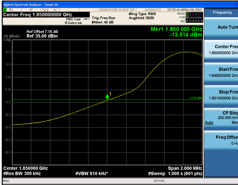
Band2-15MHz-QPSK-18675-1RB#74
