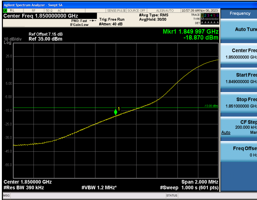
Band2-20MHz-16QAM-18700-1RB#99
