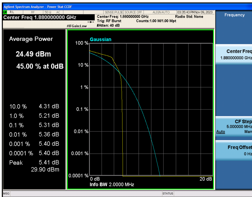
EGPRS1900-810
