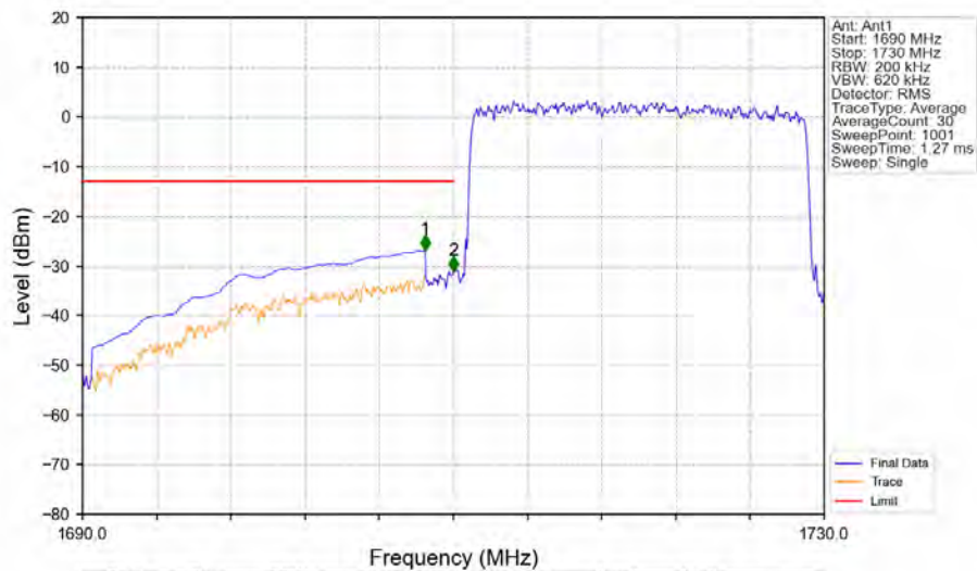
Band66_20MHz_16QAM_LCH_1720MHz_RB_100_0_NTNV
