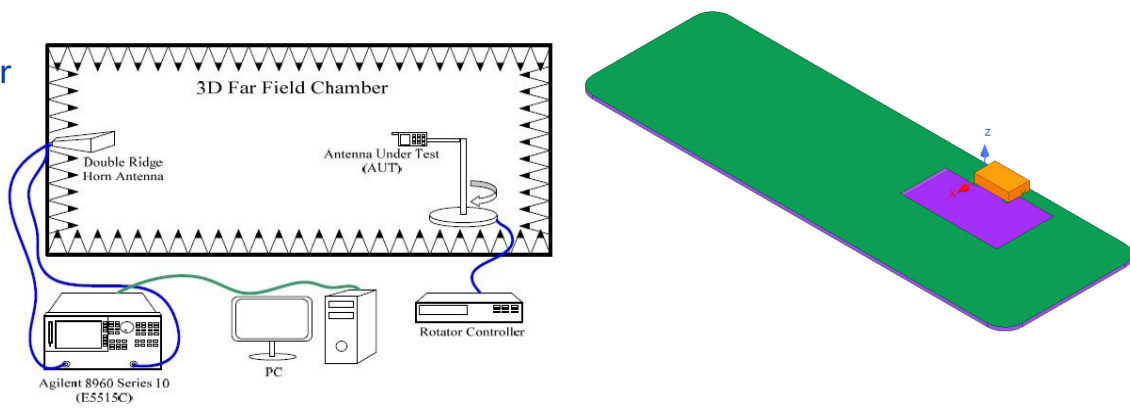
Fig.2 暗室示意图
