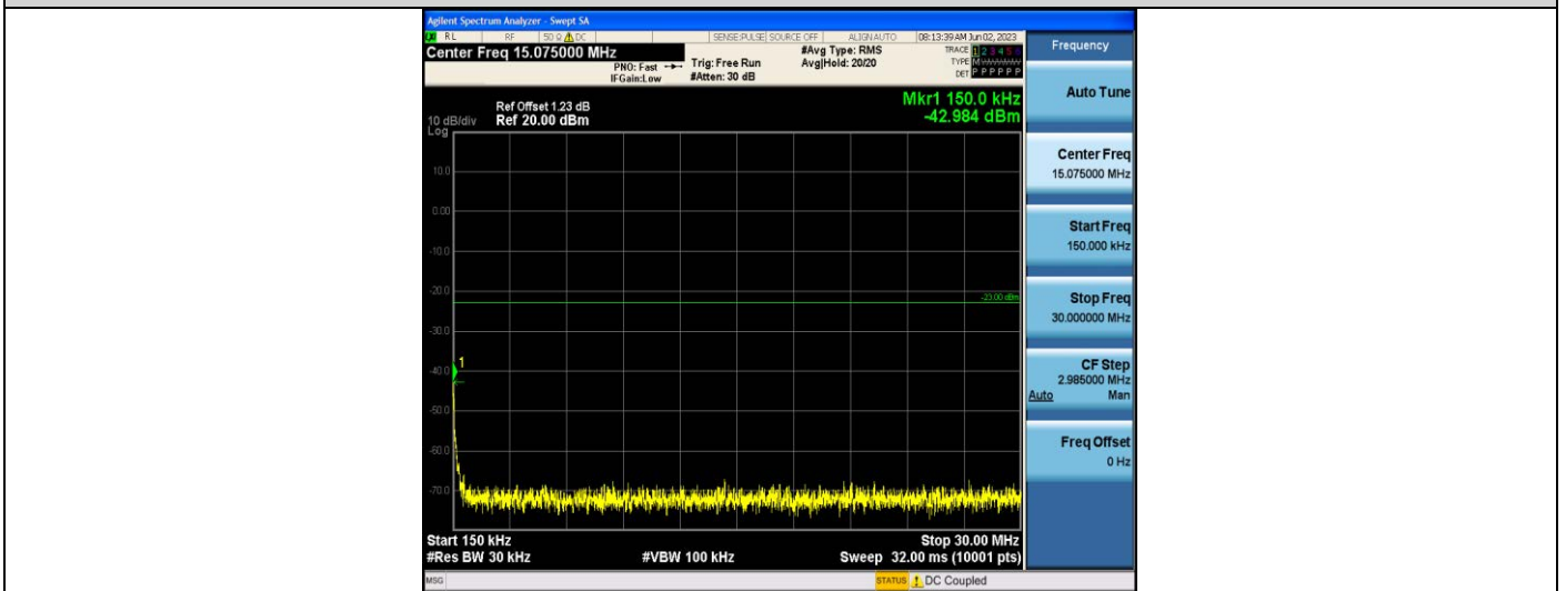
EGPRS1900-810-0.15~30MHz
