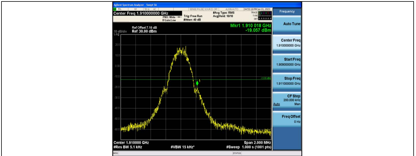
GPRS1900-512
