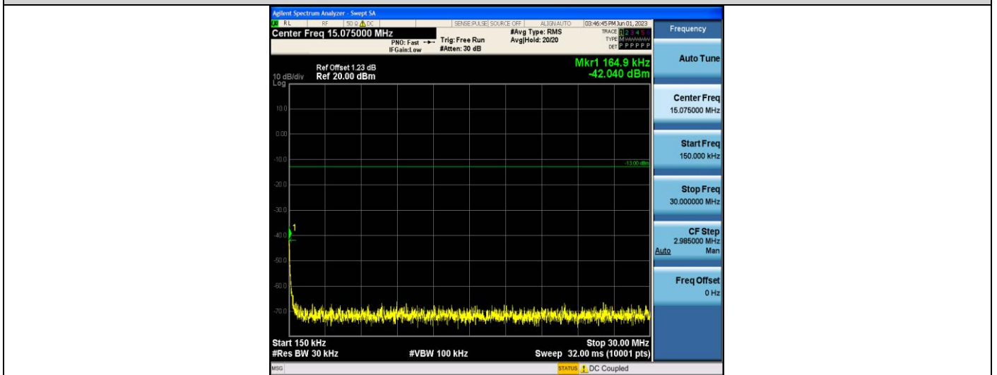
GSM850-251-0.15~30MHz
