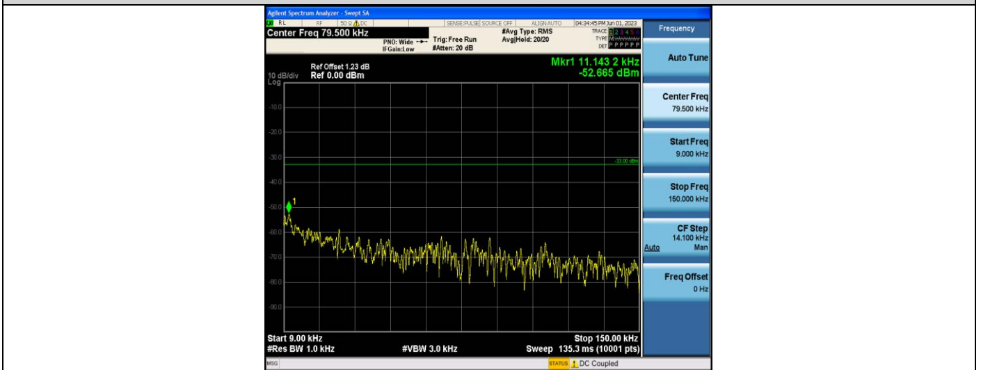
EGPRS850-128-0.009~0.15MHz
