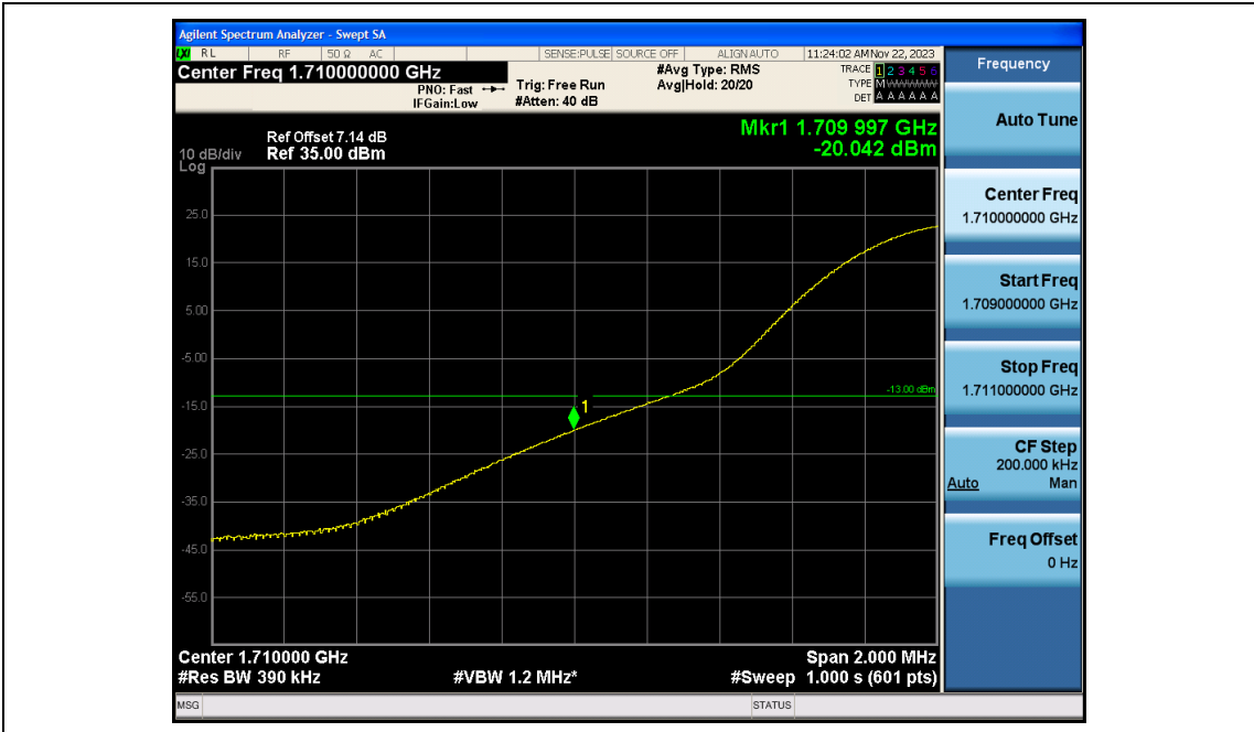
Band4-20MHz-QPSK-20050-1RB#99
