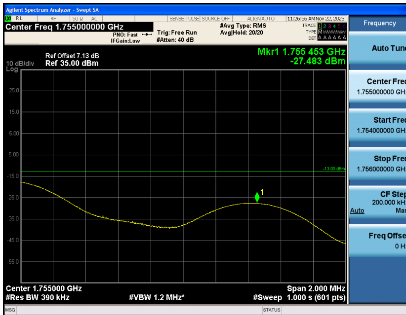
Band4-20MHz-QPSK-20300-1RB#99
