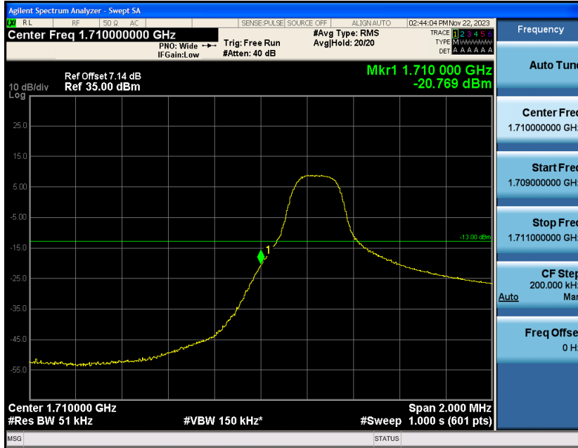
Band4-3MHz-QPSK-19965-1RB#14
