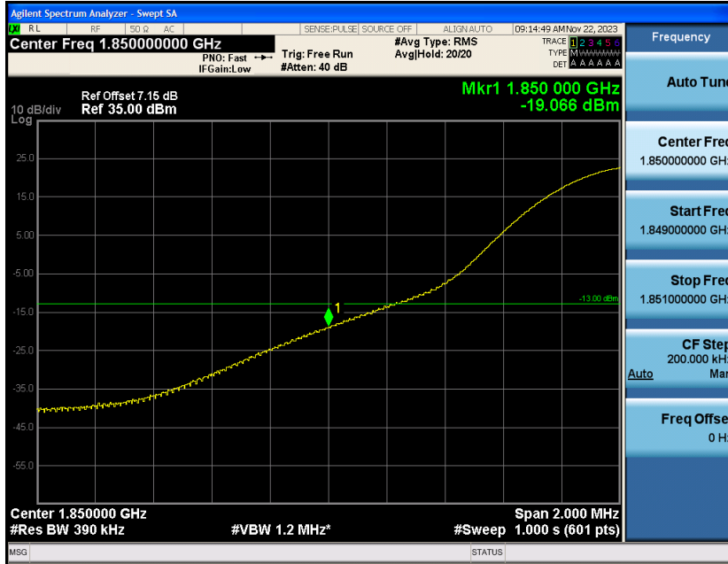
Band2-20MHz-16QAM-18700-1RB#99
