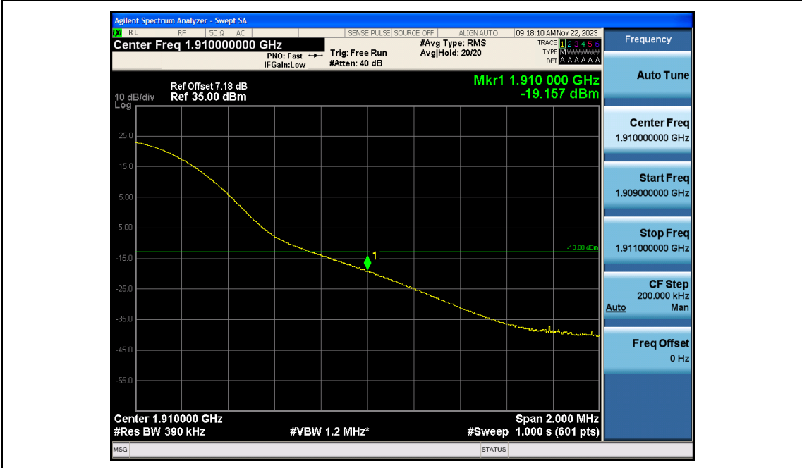
Band2-20MHz-QPSK-19100-100RB#0
