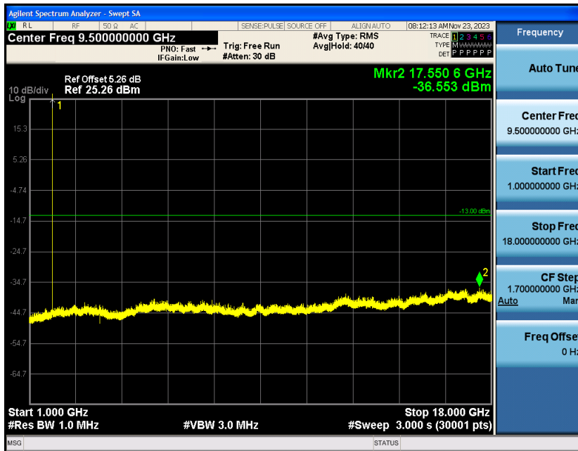
GPRS1900-661-0.009~0.15MHz
