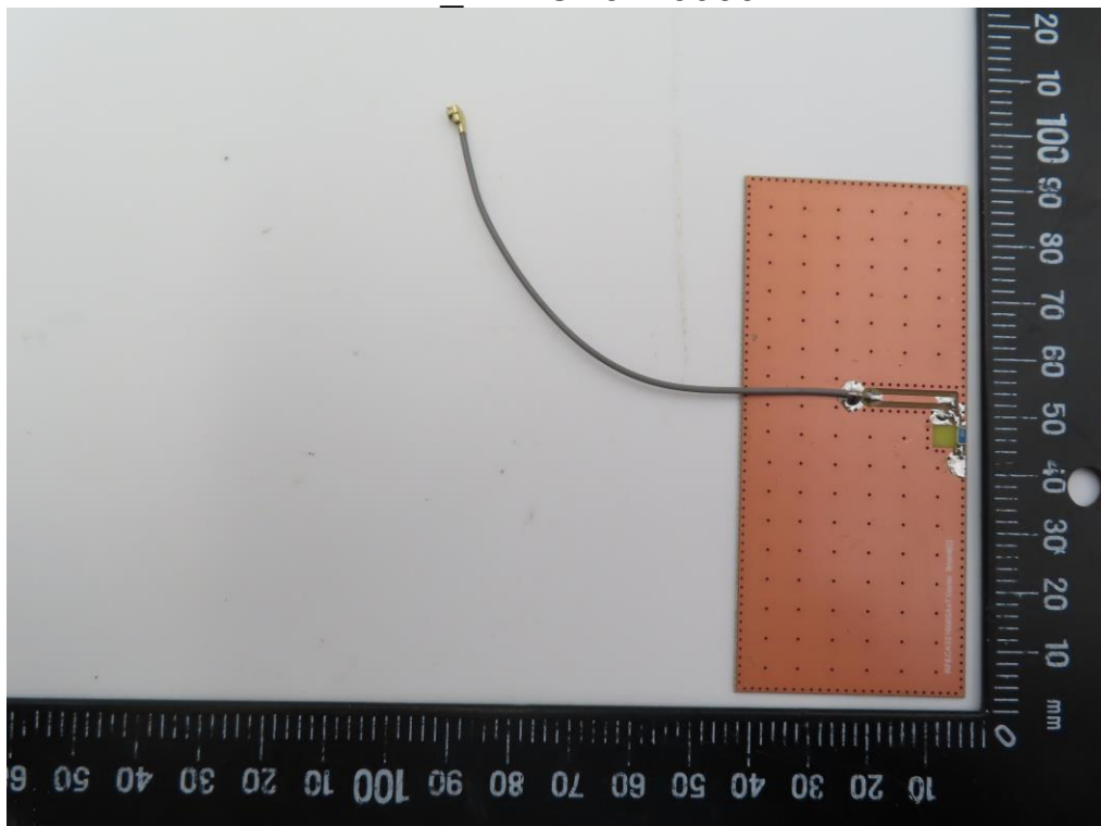
Antenna_RFDPA131010EMAB301
